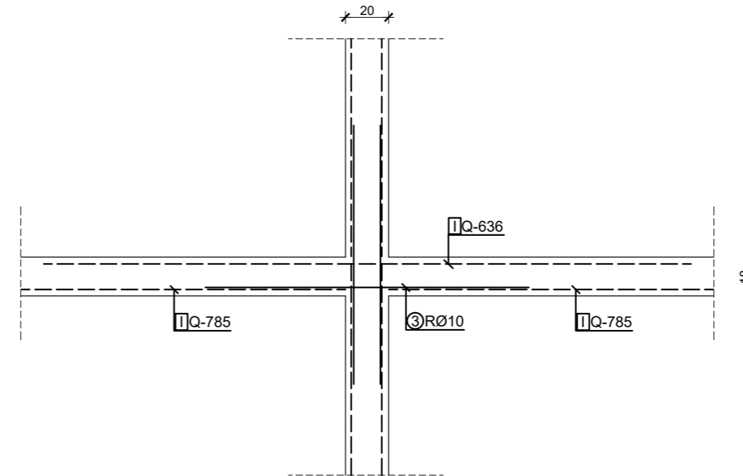
Presjke 2-2 M 1:25
