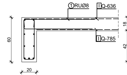
Presjke 1-1 M 1:25
