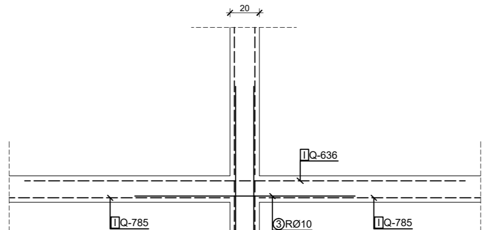
Presjke 2-2 M 1:25
