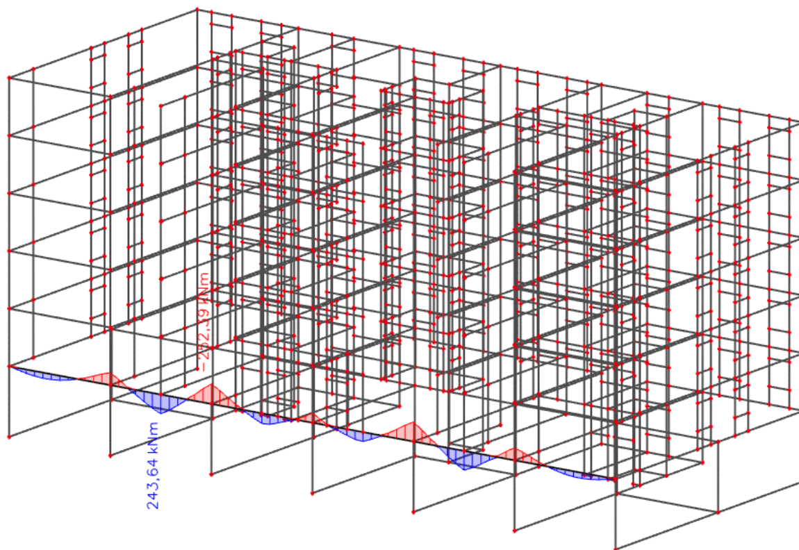
Slika 9.7 Moment savijanja M_{Ed,y} (kNm) za GSN-1
