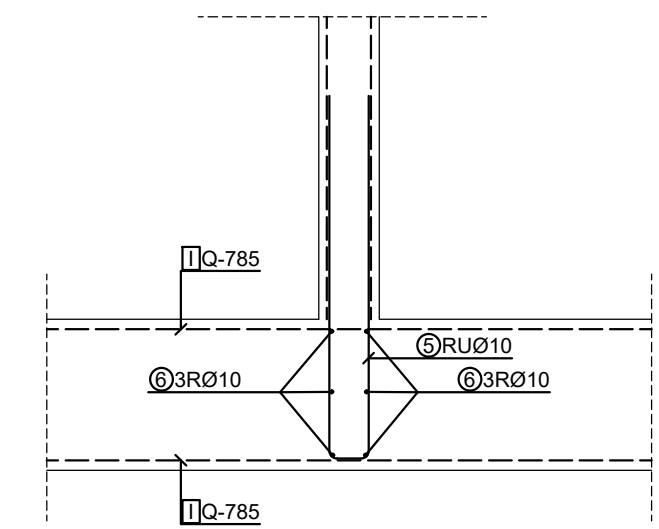
Presjke 2-2 M 1:25
