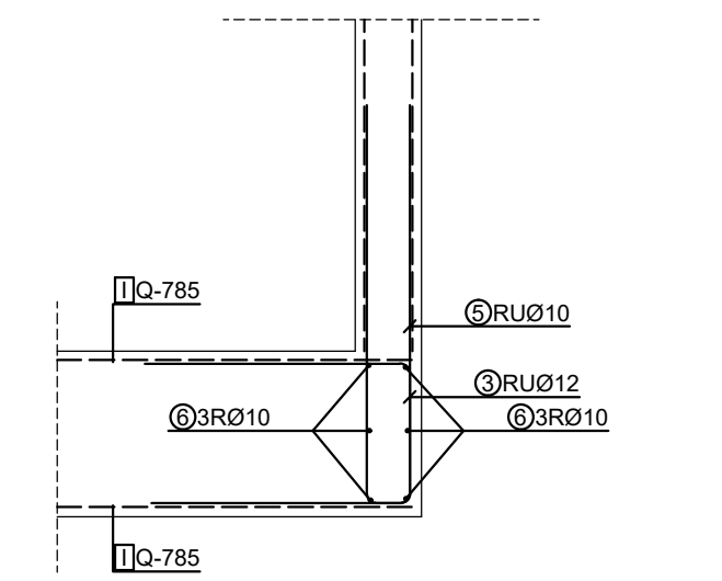
Presjke 2-2 M 1:25
