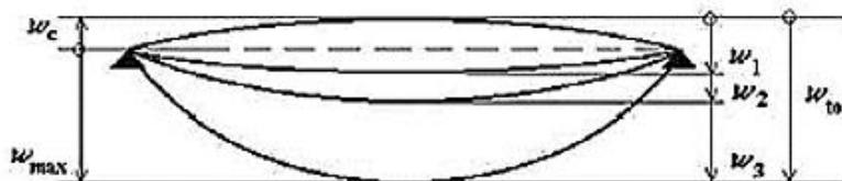
Slika 6.7 Prikaz progiba ploča
