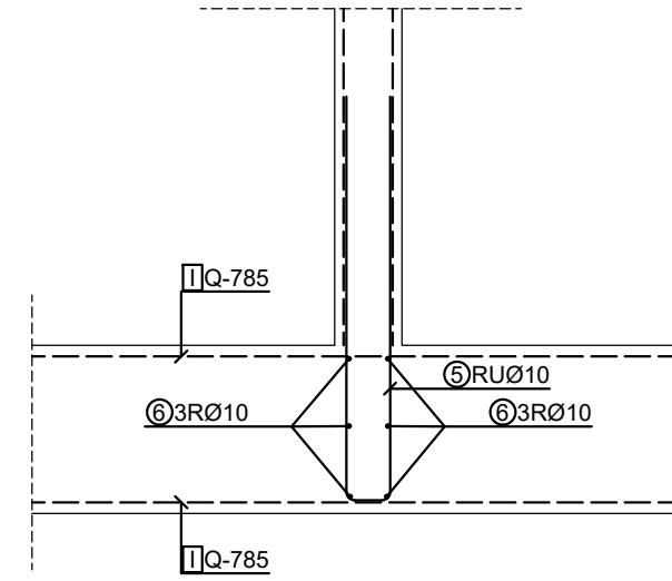
Presjke 2-2 M 1:25
