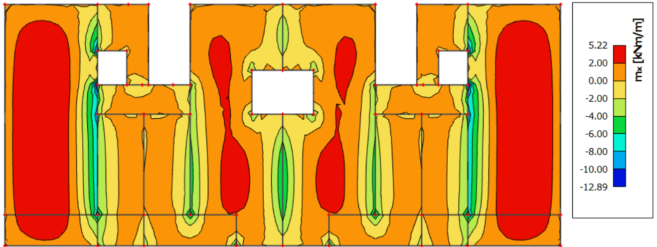
Slika 7.5 Armatura u međukatnoj ploči smjer A_{s,x-x} ( \text{cm}^2/\text{m} ) za GSN-1
