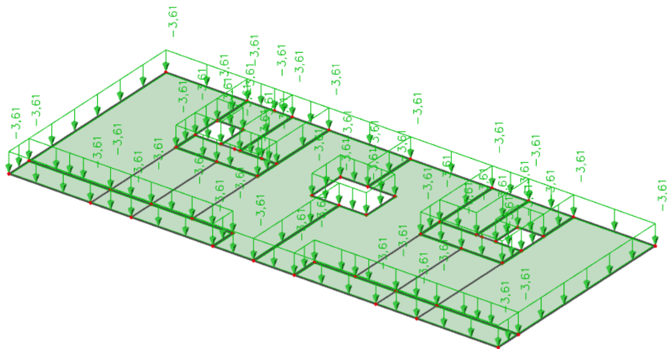
Slika 4.7 Dodatno stalno djelovanje \Delta g ( \text{kN/m}^2 )
