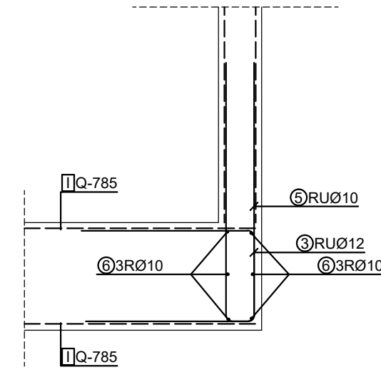
Presjke 2-2 M 1:25
