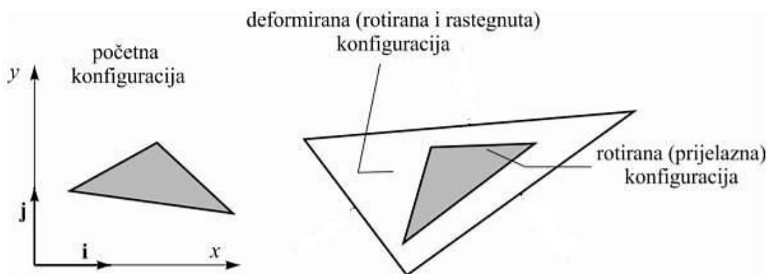
Slika 4.10. Prikaz pomaka trokutastog elementa [17].
