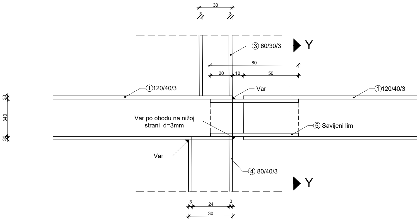
Detalj D 2 1:2
