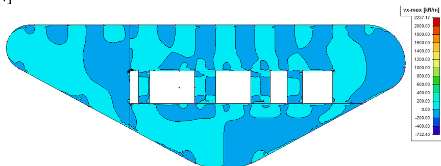
Slika 5.4. Poprečna sila v_x
