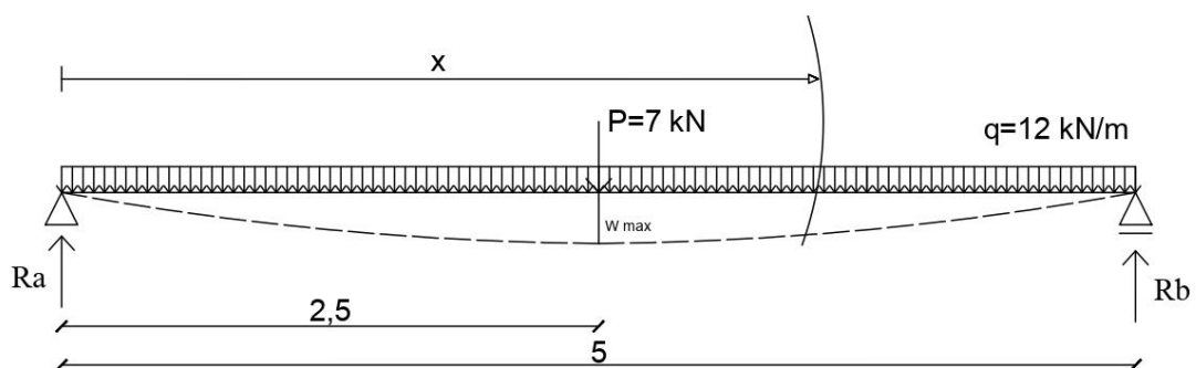
Slika 5. Prikaz analiziranog nosača
