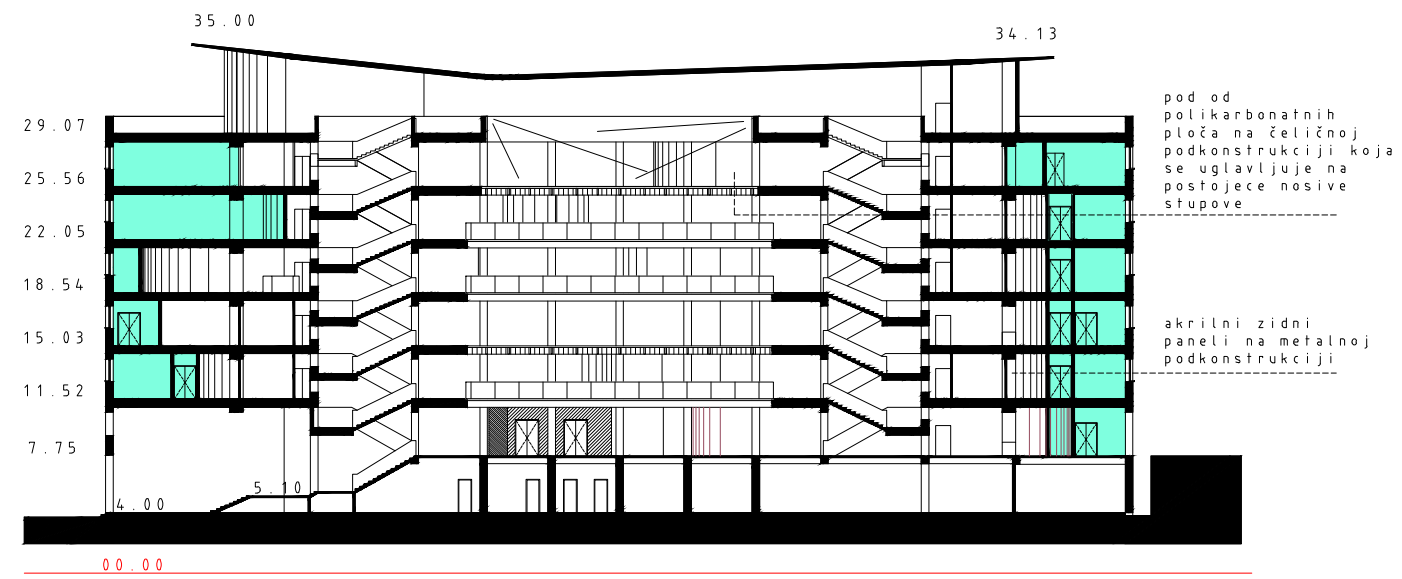
presjek A-A
