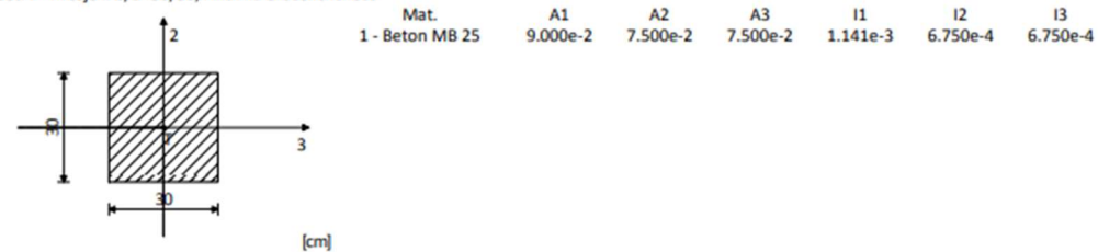
Set: 7 Presjek: b/d=30/30 , Fiktivna ekscentričnost
