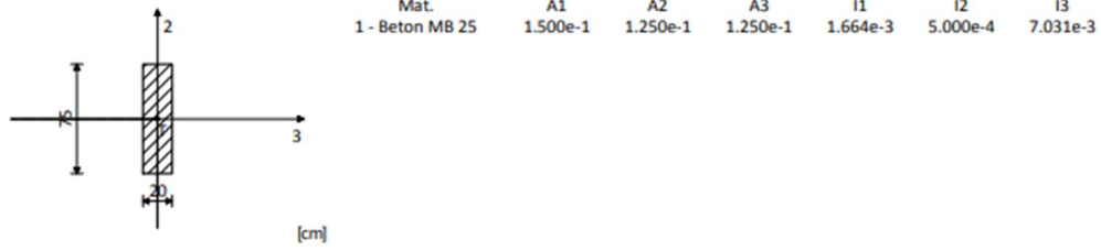
Set: 1 Presjek: b/d=20/75 , Fiktivna ekscentričnost
