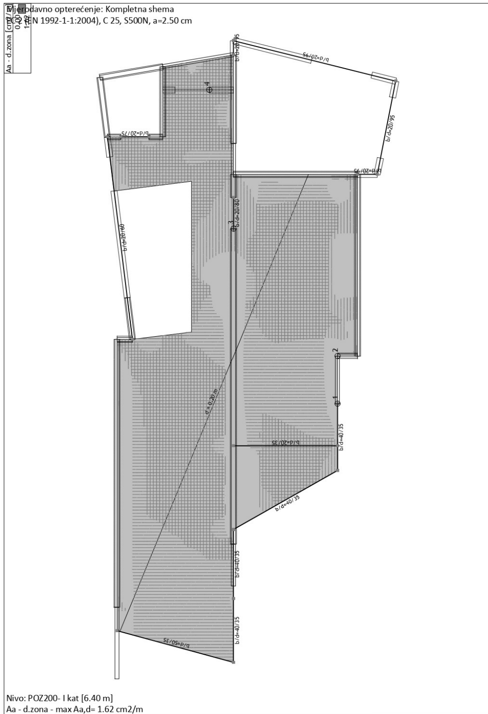
Slika 81. Potrebna armatura za donju zonu ploče POZ200
