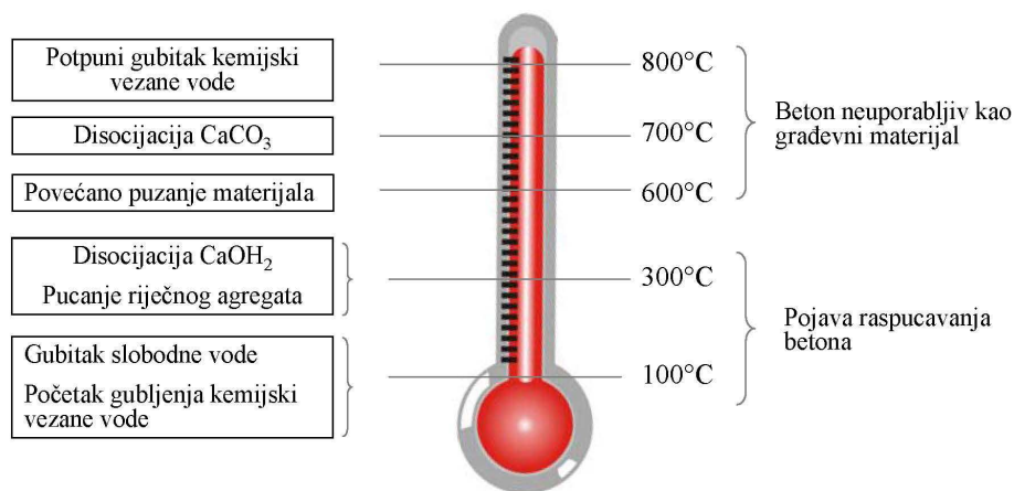
Crtež 5.3. Stadiji temperaturno ovisnih kemijskih promjena u betonu
