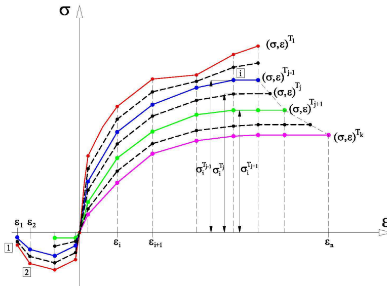
Crtež 4.5. Interpolacija nelinearne veze naprežanje-deformacija (\sigma, \varepsilon)^{T_j} za temperaturu T_j između dvije poznate veze naprežanje-deformacija za temperature T_{j-1} i T_{j+1}
