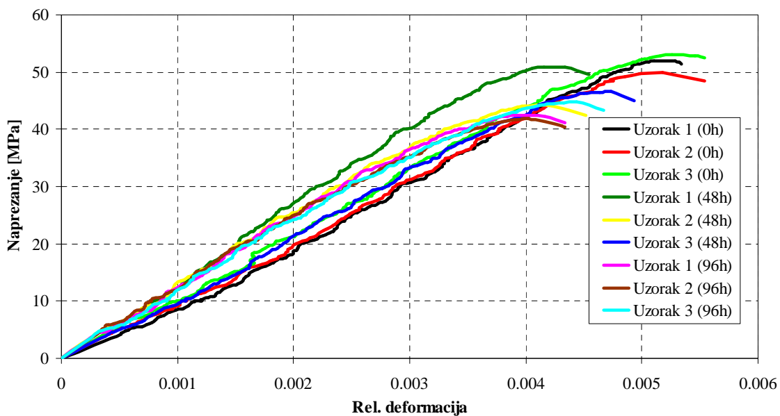
Grafikon 5.20. Usporedbe krivulja napreznaje-deformacija - 400°C (0-96h)
