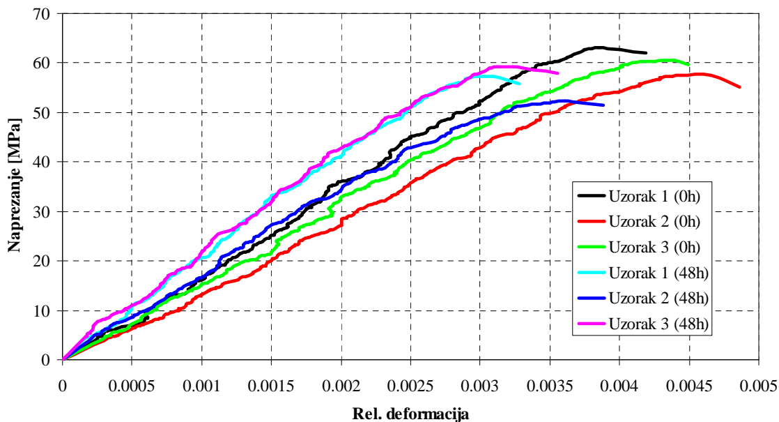
Grafikon 5.19. Usporedbe krivulja napreznaje-deformacija - 230°C (0-48h)
