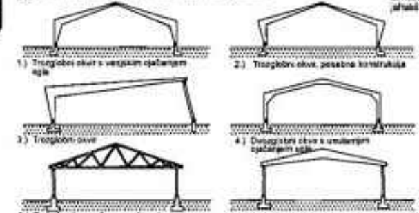
3 Poprečni presjeci hala
