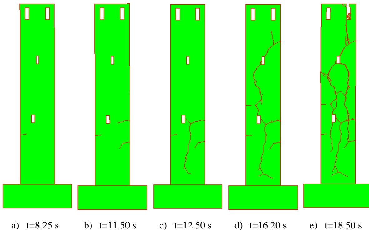
Pojava i širenje pukotina za vršno ubrzanje 0.40 g
