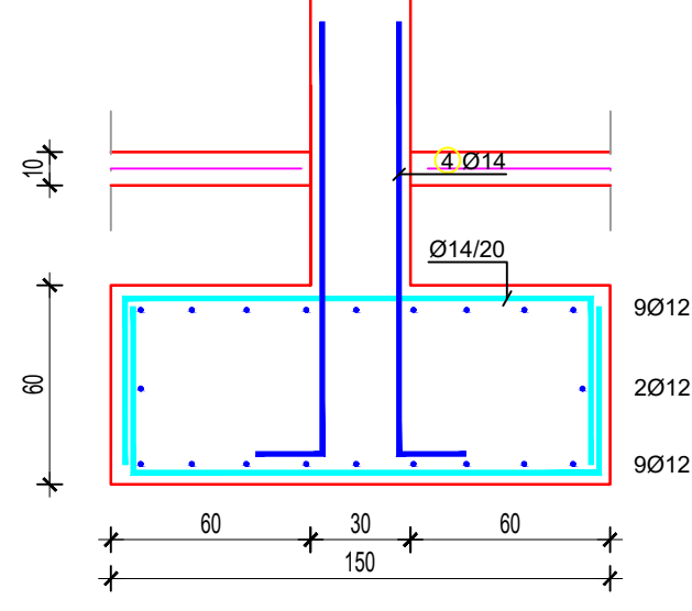
Presjek 2-2 R=1:25
