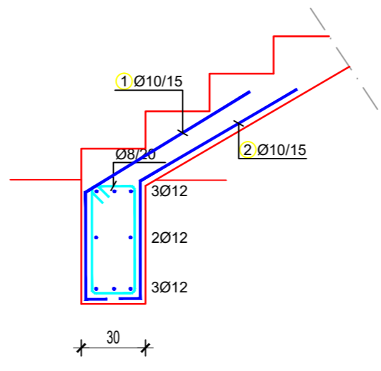
Presjek 3-3 R=1:25
