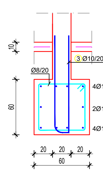
Presjek 1-1 R=1:25
