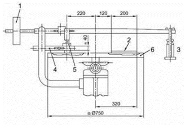
Slika 4.4. Uređaj za ispitivanje habanja [16]
