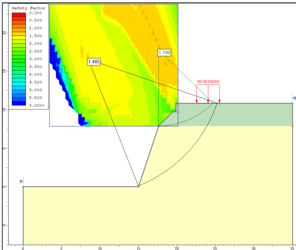
Slika 19. Prikaz rezultata za osnovnu proračunsku kombinaciju za presjek 1-1 (sjever)
