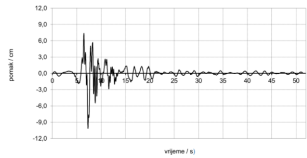
Slika 38. Pomaci nastali ubrzanjem podloge
