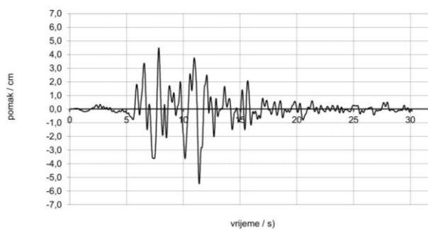
c) vršno ubrzanje 0.15 g
