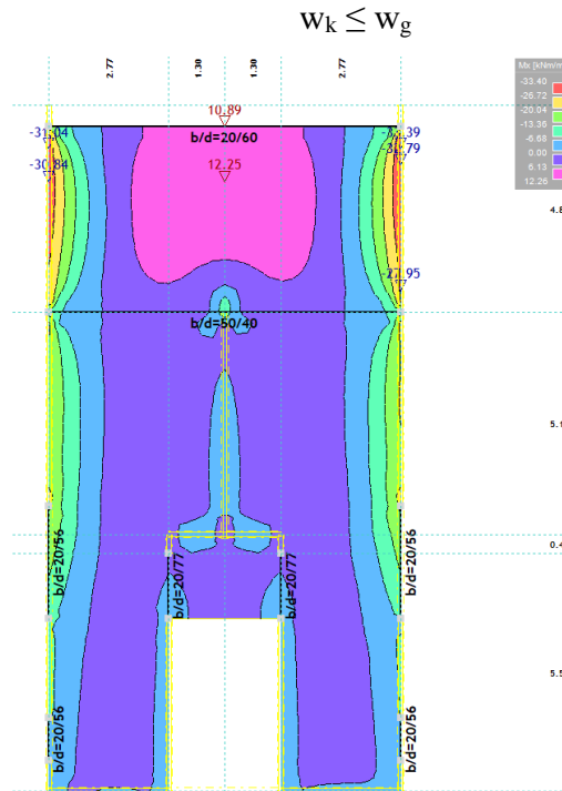
Slika 11.18. Moment savijanja M_x - GSU
