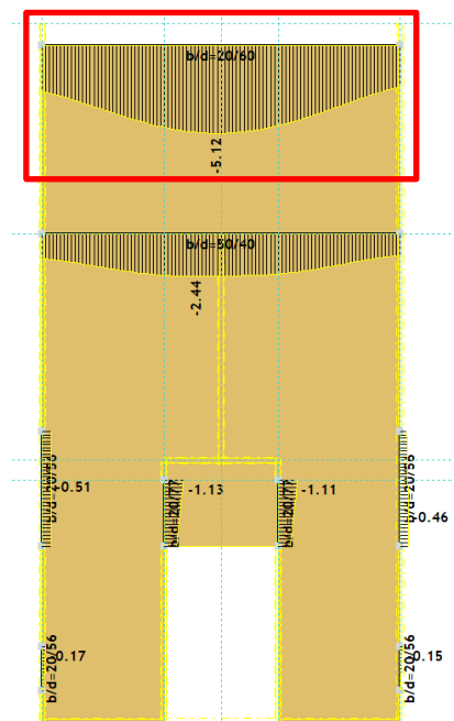
Slika 12.10. Prikaz progiba grede G201- GSU
