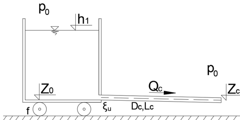
Slika 1. Vodospremnik s ispuštom
