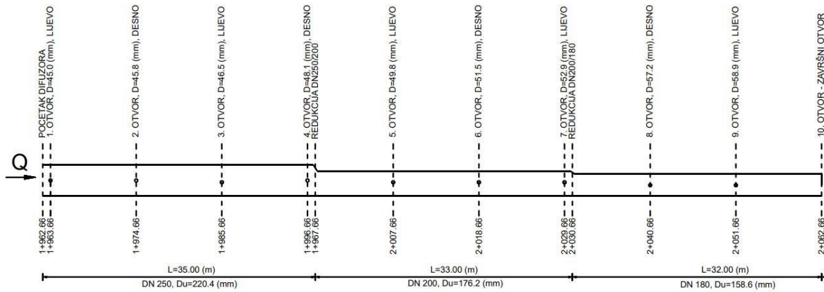
Slika 2.4. Shematski prikaz dionica difuzora [1]
