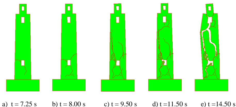
Slika 172. Širenje i nastanak pukotina za vršno ubrzanje \mathbf{a}_g = 0.35 g za Petrovac, potpuni slom
