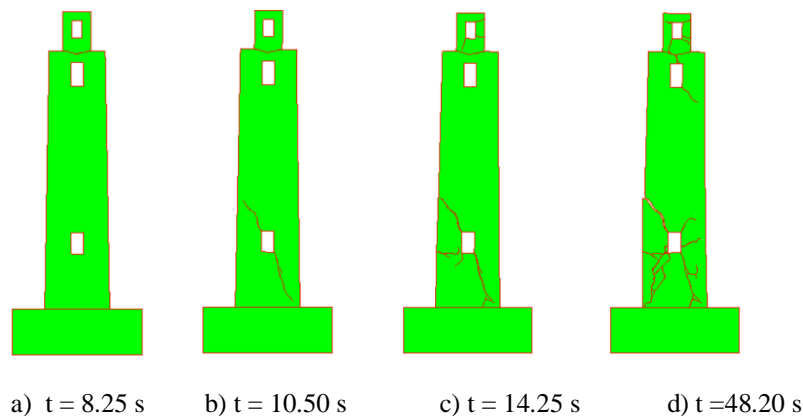
Slika 171. Širenje i nastanak pukotina za vršno ubrzanje a_g = 0.33 g za Petrovac
