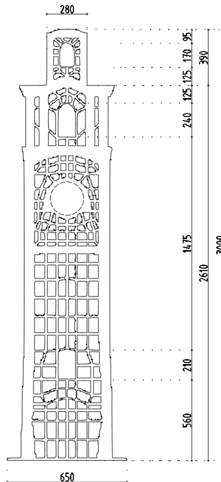
Slika 9. Geometrijski model konstrukcije.
