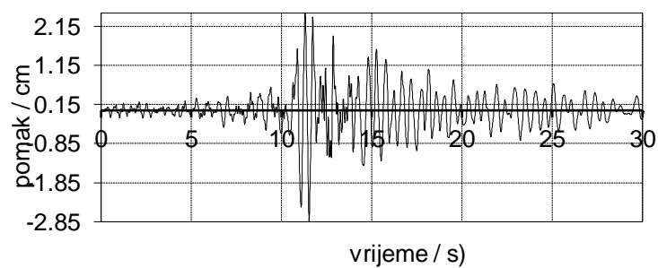
Slika 77. Vršno ubrzanje a_g = 1.20 g za Campano Lucano
