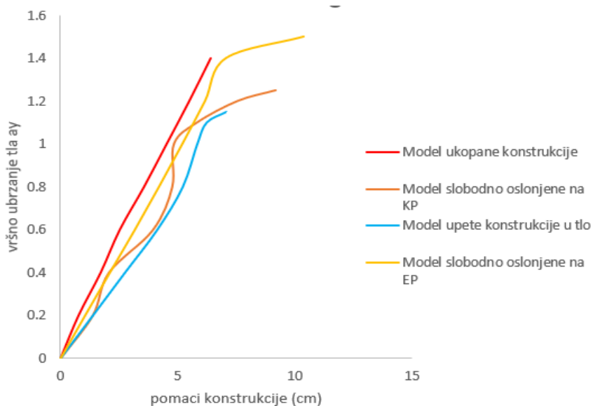
Slika 198. Pomaci vrha konstrukcije za South Iceland
