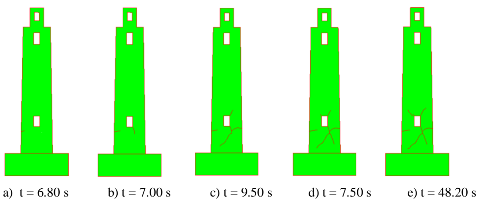
Slika 155. Širenje i nastanak pukotina za vršno ubrzanje a_g = 0.25 g za Petrovac
