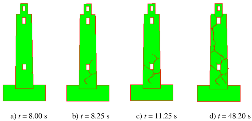
Slika 191. Širenje i nastanak pukotina za vršno ubrzanje \alpha_g = 0.46 g za Petrovac
