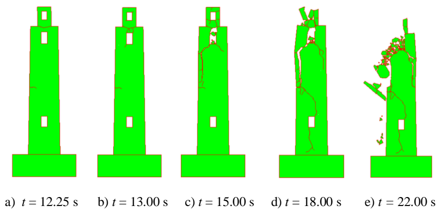
Slika 128. Širenje i nastanak pukotina za vršno ubrzanje a_g = 3.30 g za Campano Lucano
