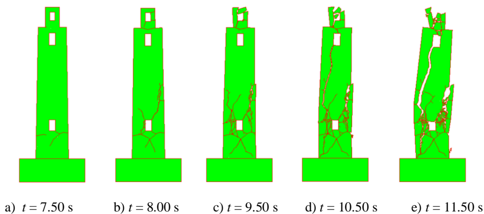
Slika 153. Širenje i nastanak pukotina za vršno ubrzanje \mathbf{a}_g = 1.50 g za South Iceland, potpuni slom
