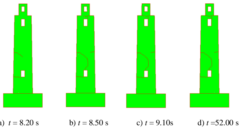
Slika 166. Širenje i nastanak pukotina za vršno ubrzanje \mathbf{a}_g = 1.10 g za South Iceland
