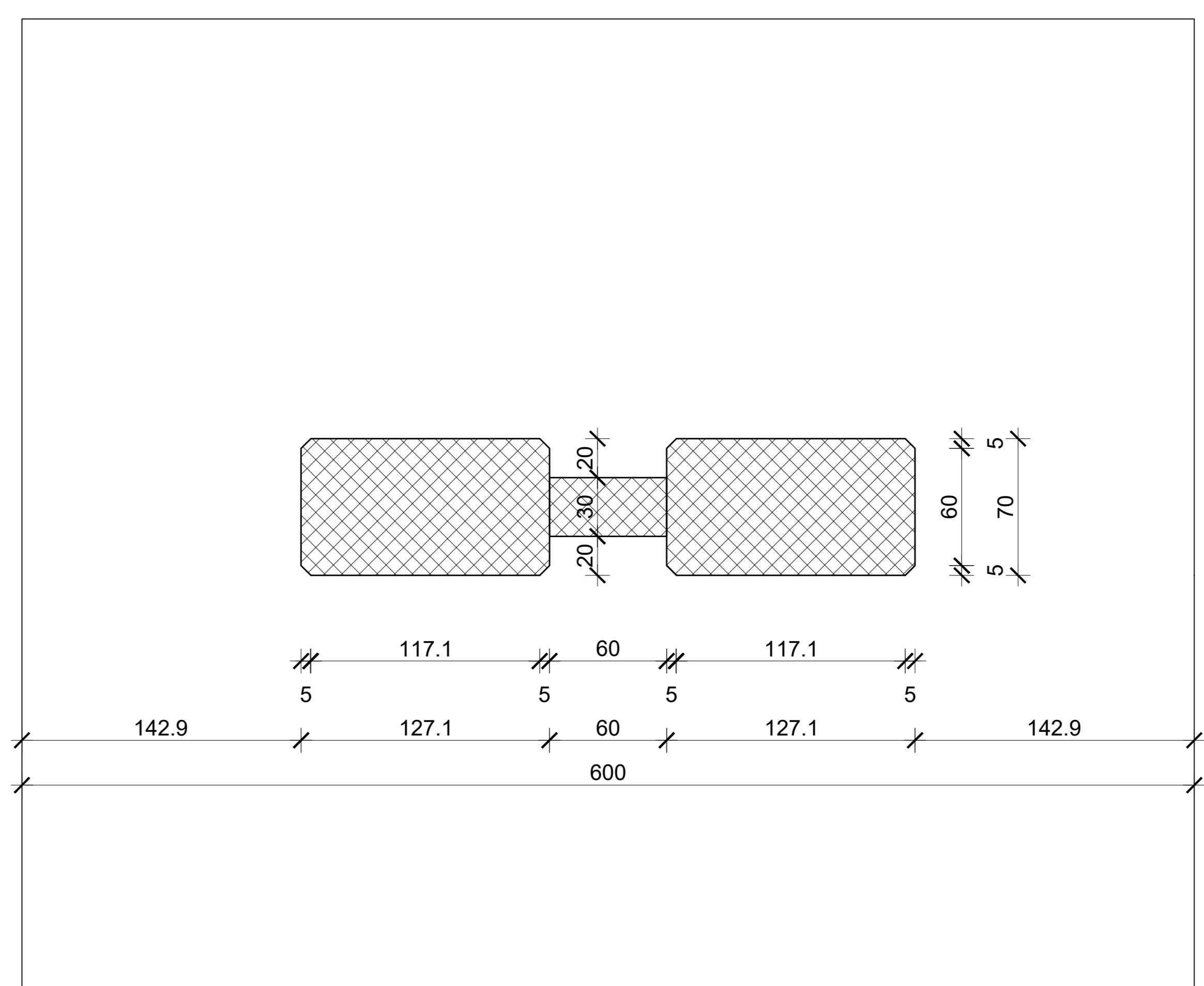
Presjek 4-4
