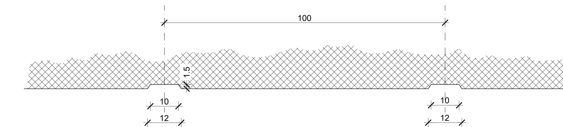
Detalj drenage
