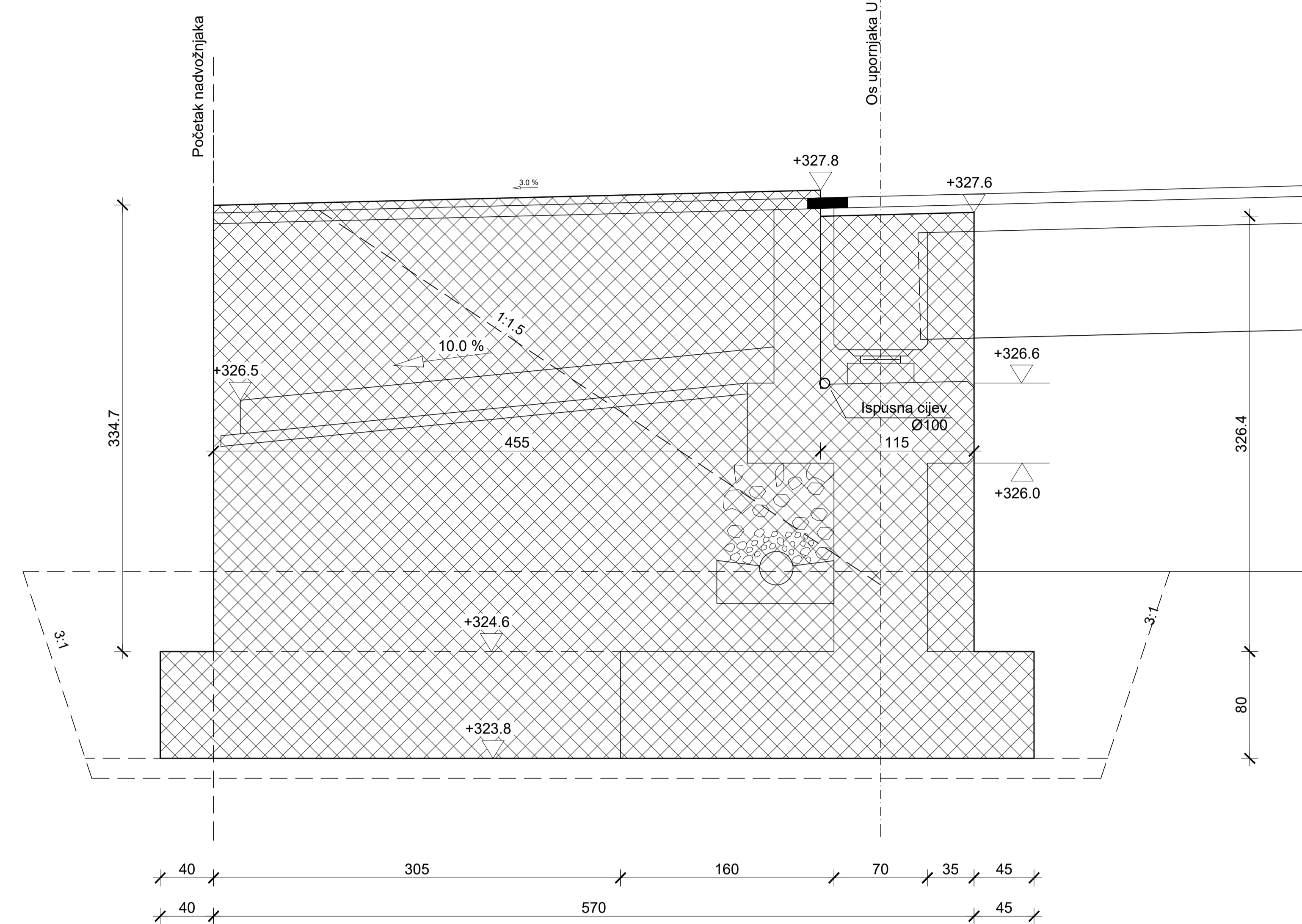
Presjek 6-6
