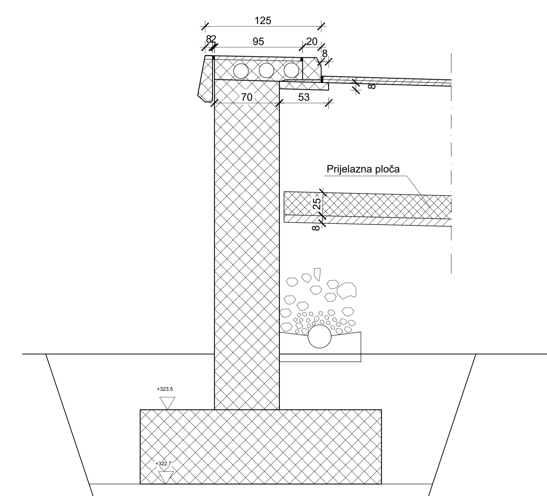
Presjek 7-7
