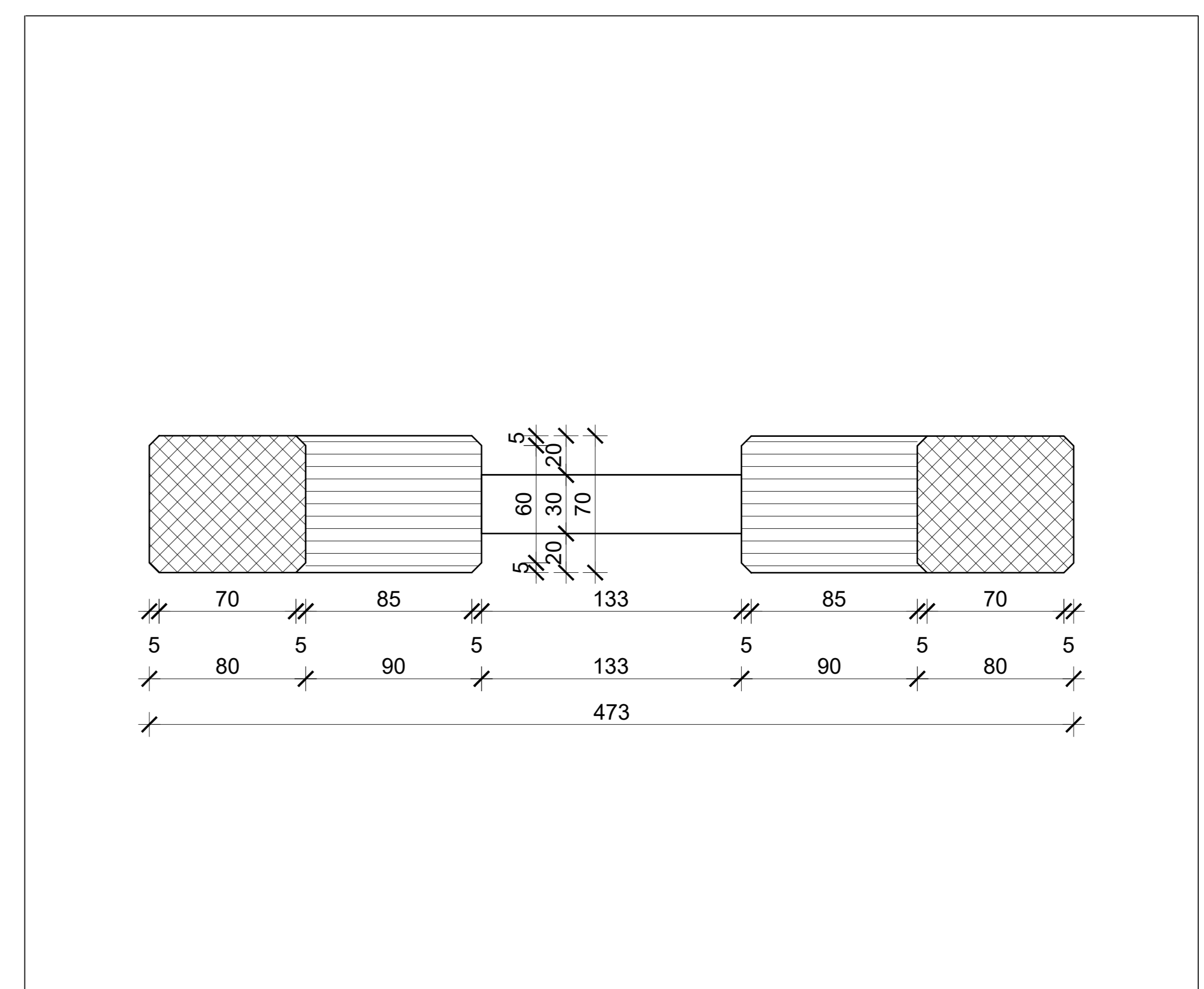
Presjek 4-4
