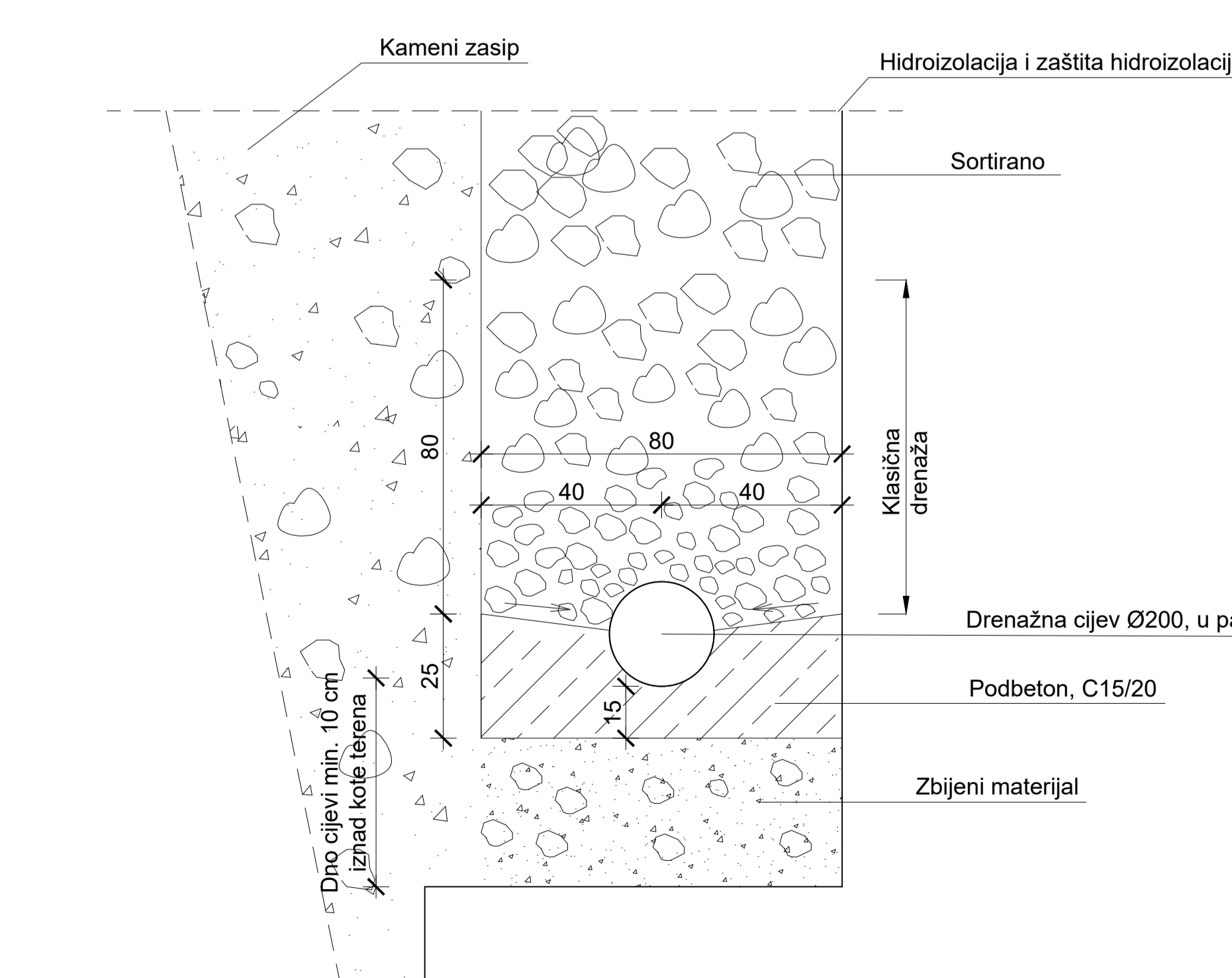
Detalj drenáže
