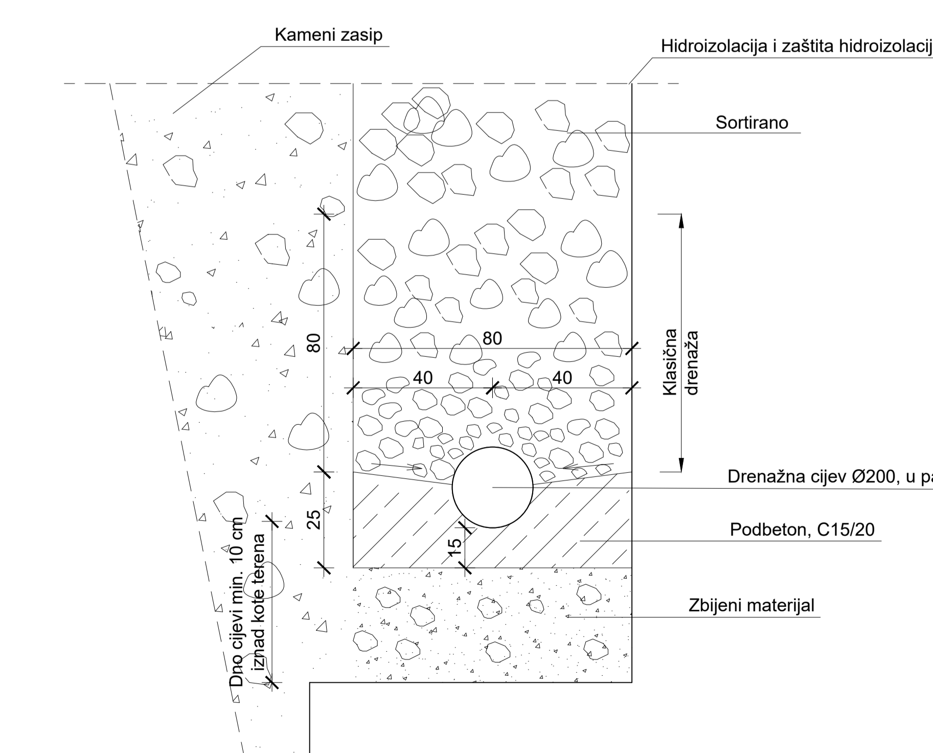
Detalj drenage
