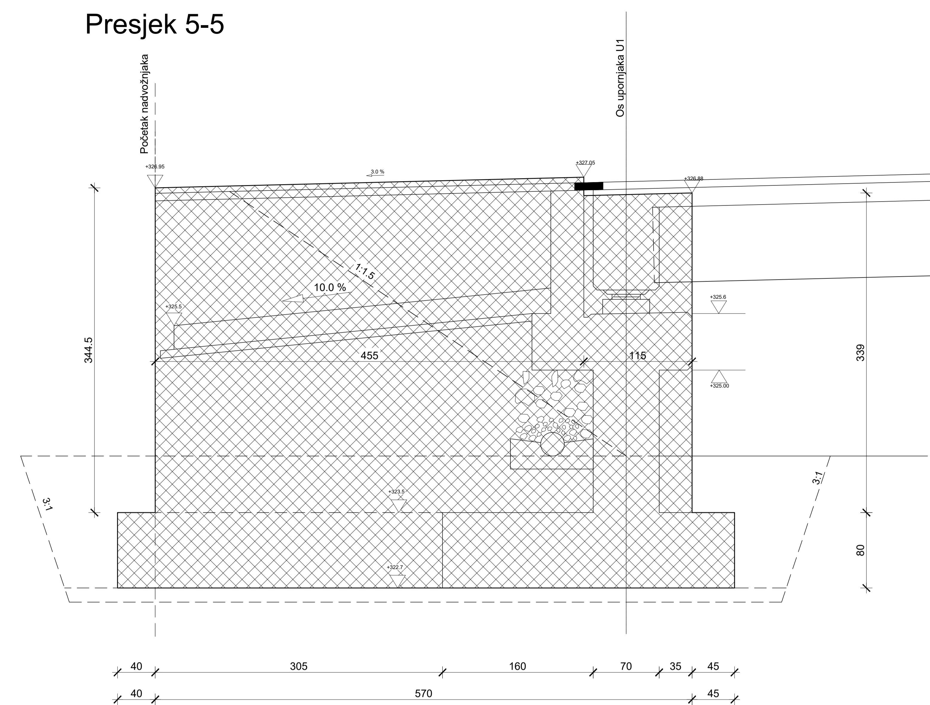
Presjek 5-5
