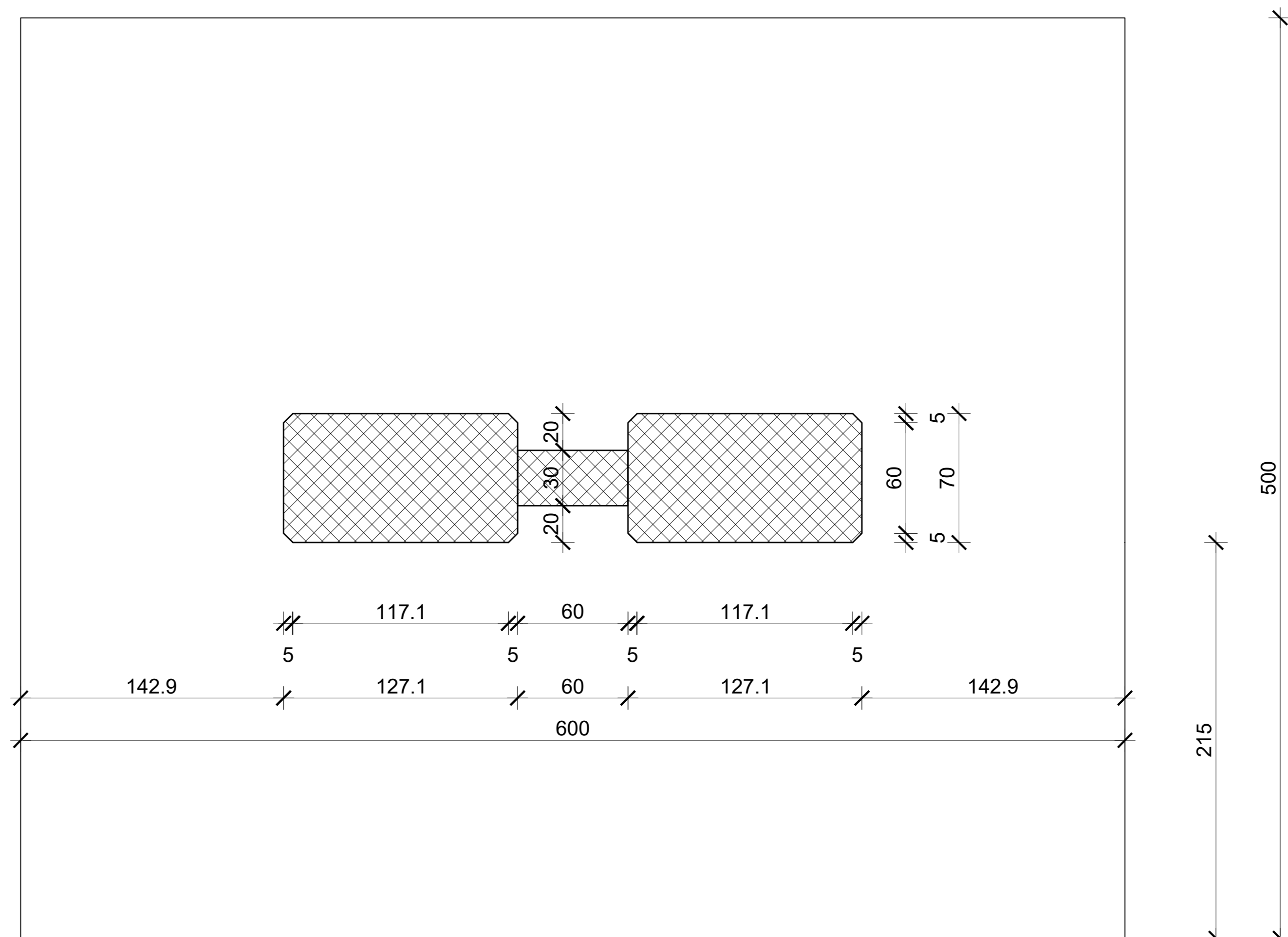
Presjek 4-4
