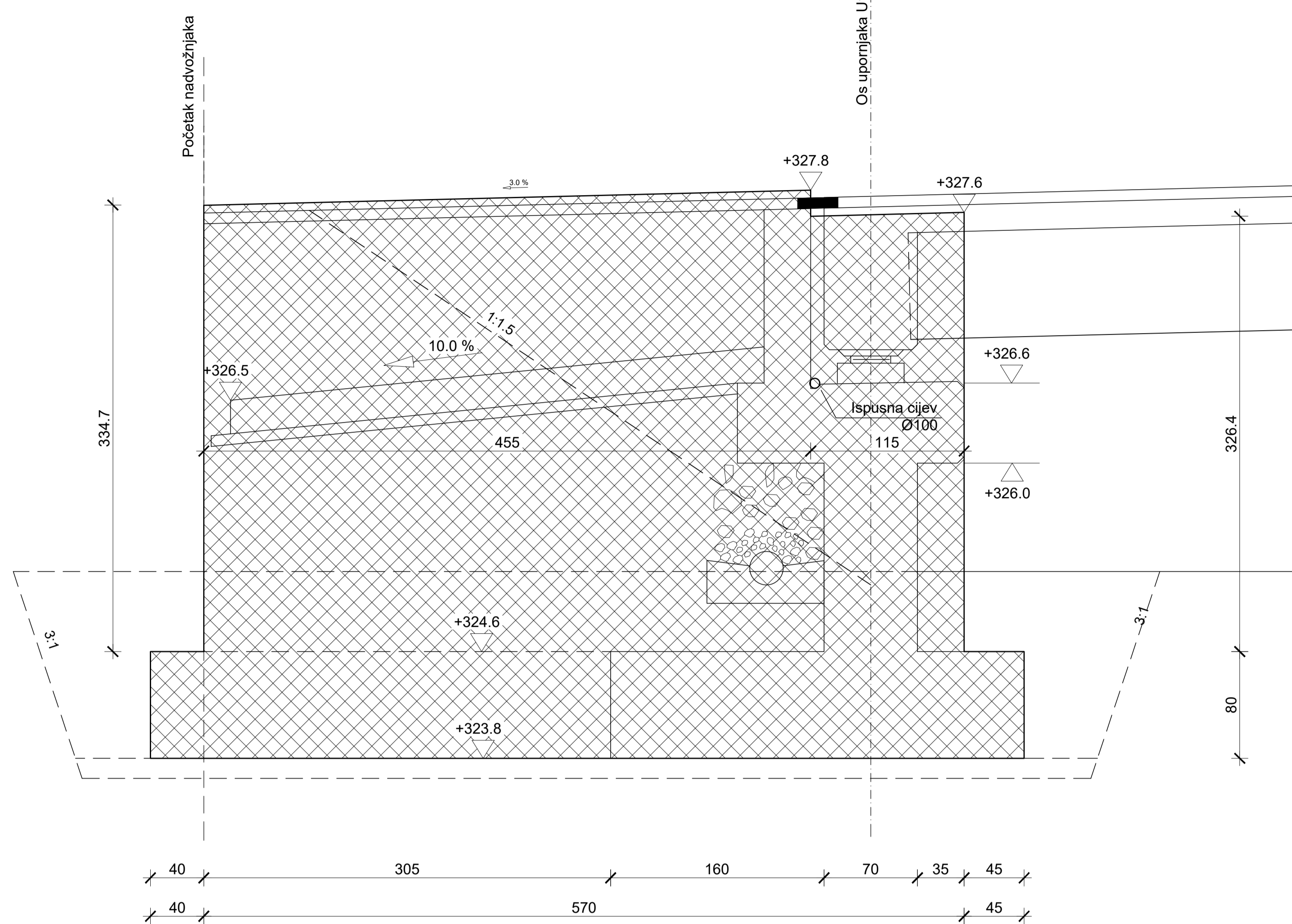
Presjek 6-6
