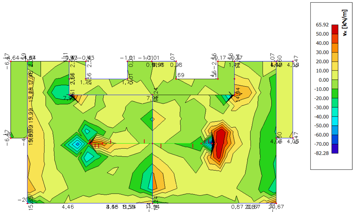
Slika 6.5 Poprečne sile V_{Ed,x} (kN/m) za GSN-1
