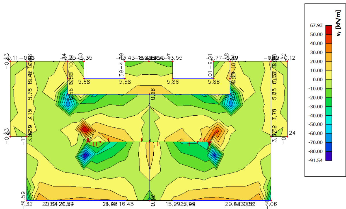
Slika 6.6 Poprečne sile V_{Ed,y} (kN/m) za GSN-1
