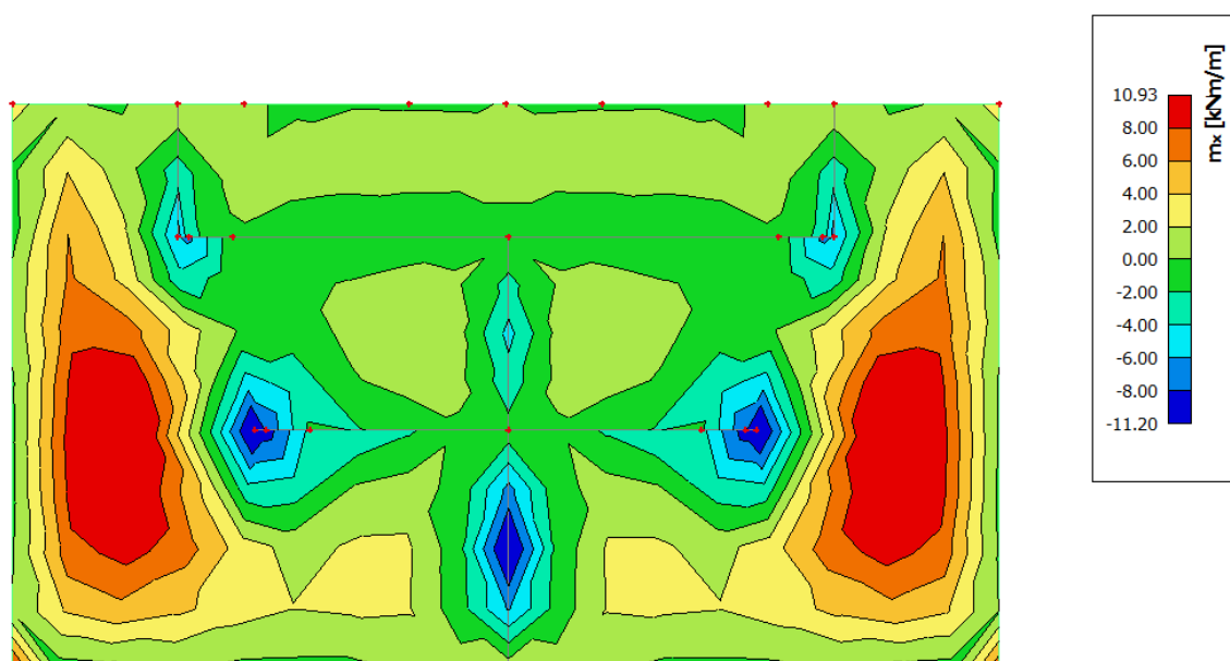
Slika 6.23 Moment savijanja M_{Ed,x} (kNm/m) za GSU-1
