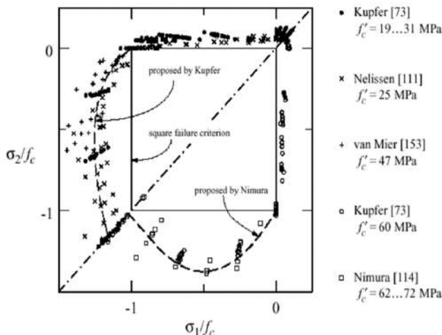
Slika 2.5 – Tzv. Kupferov test – dvoosno stanje naprežanja u betonu
