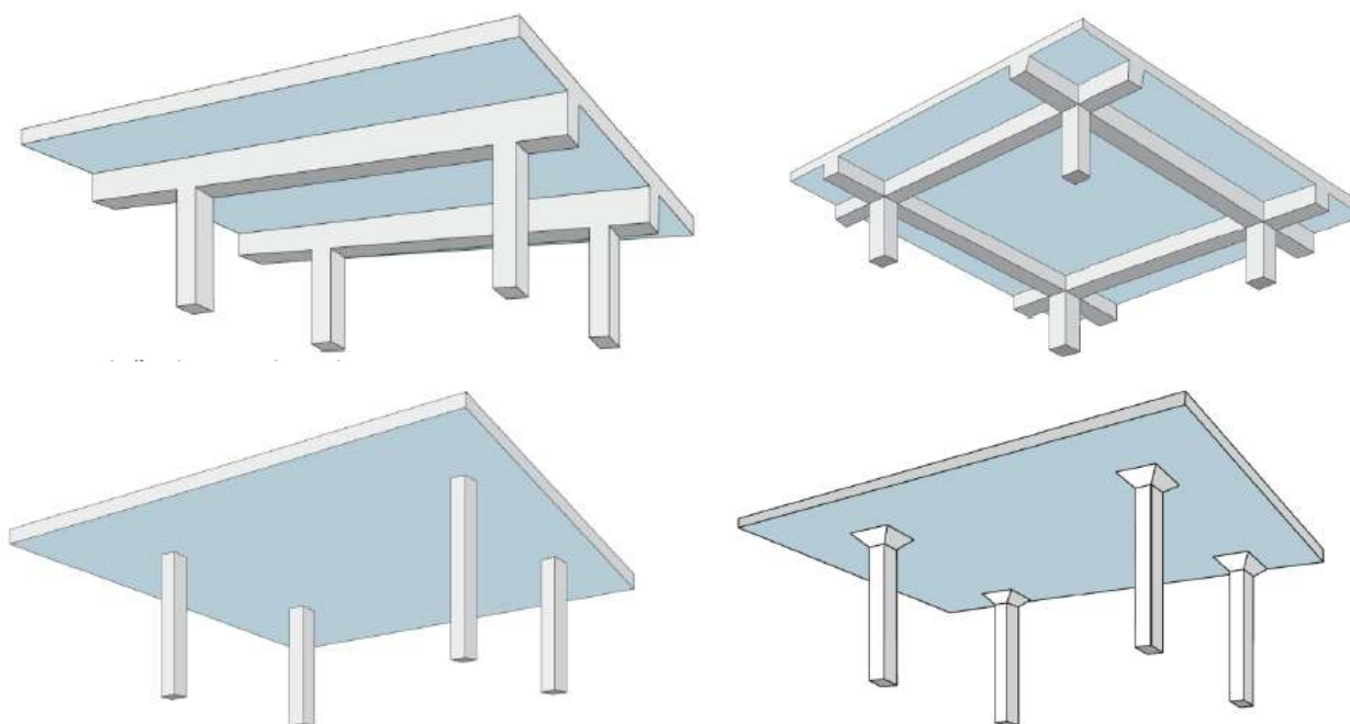
Slika 6.3 – Načini oslanjanja ploča: Oslanjanje na grede (gornje slike); oslanjanje na stupove (donje slike) [7]
