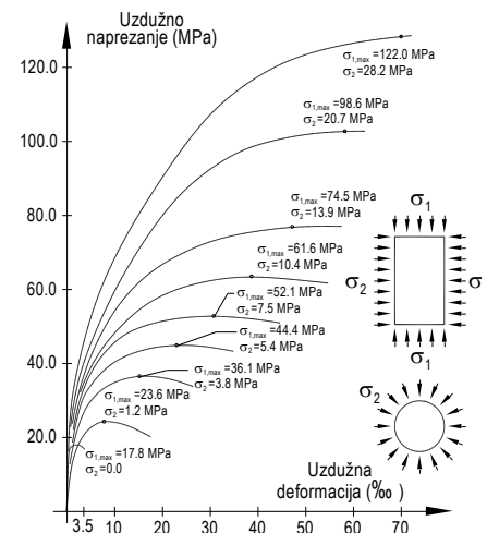
Slika 2.6 – Dijagram \sigma - \epsilon betona pri troosnom stanju naprežanja
