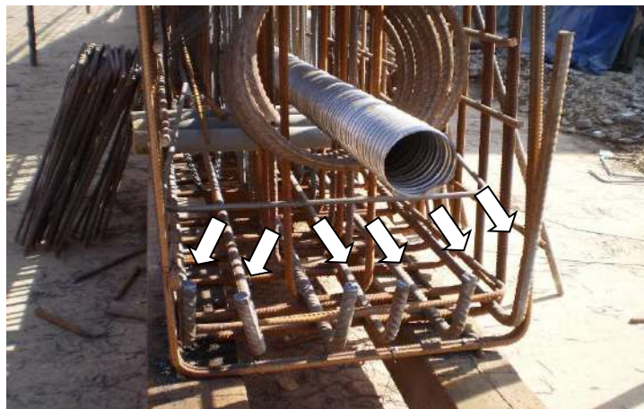
Slika 7.25 – Obična armatura postavljena u armaturnom košu djelomično prednapetog nosača
