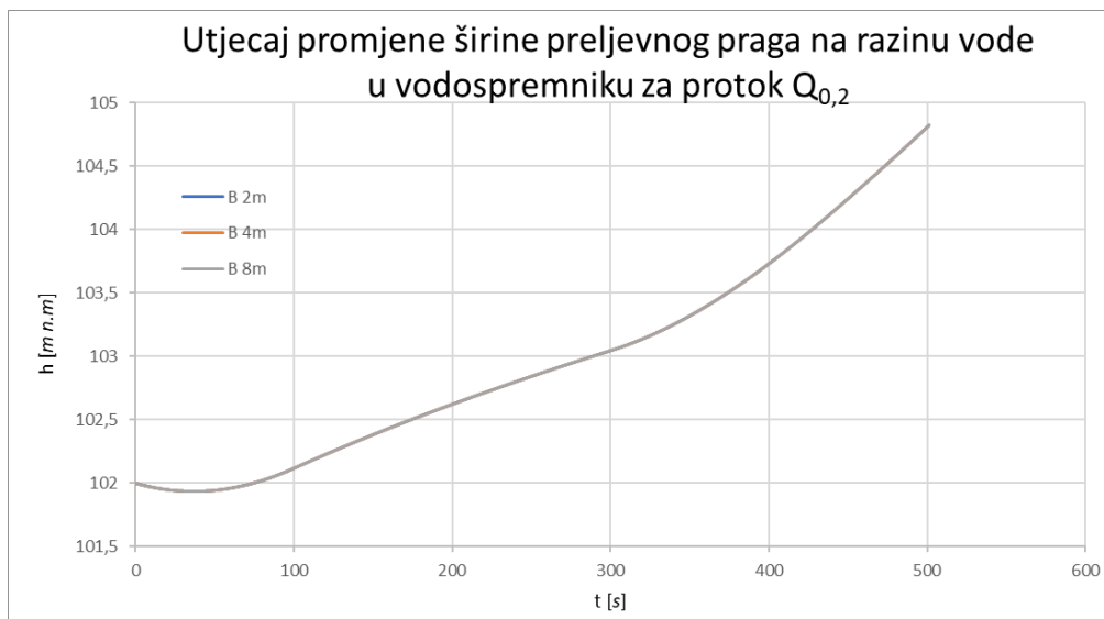
Slika 18. Utjecaj promjene širine prelijevnog praga 2 (m), 4(m), 8(m) na razinu vode u vodospremniku za protok Q_{0,2}
