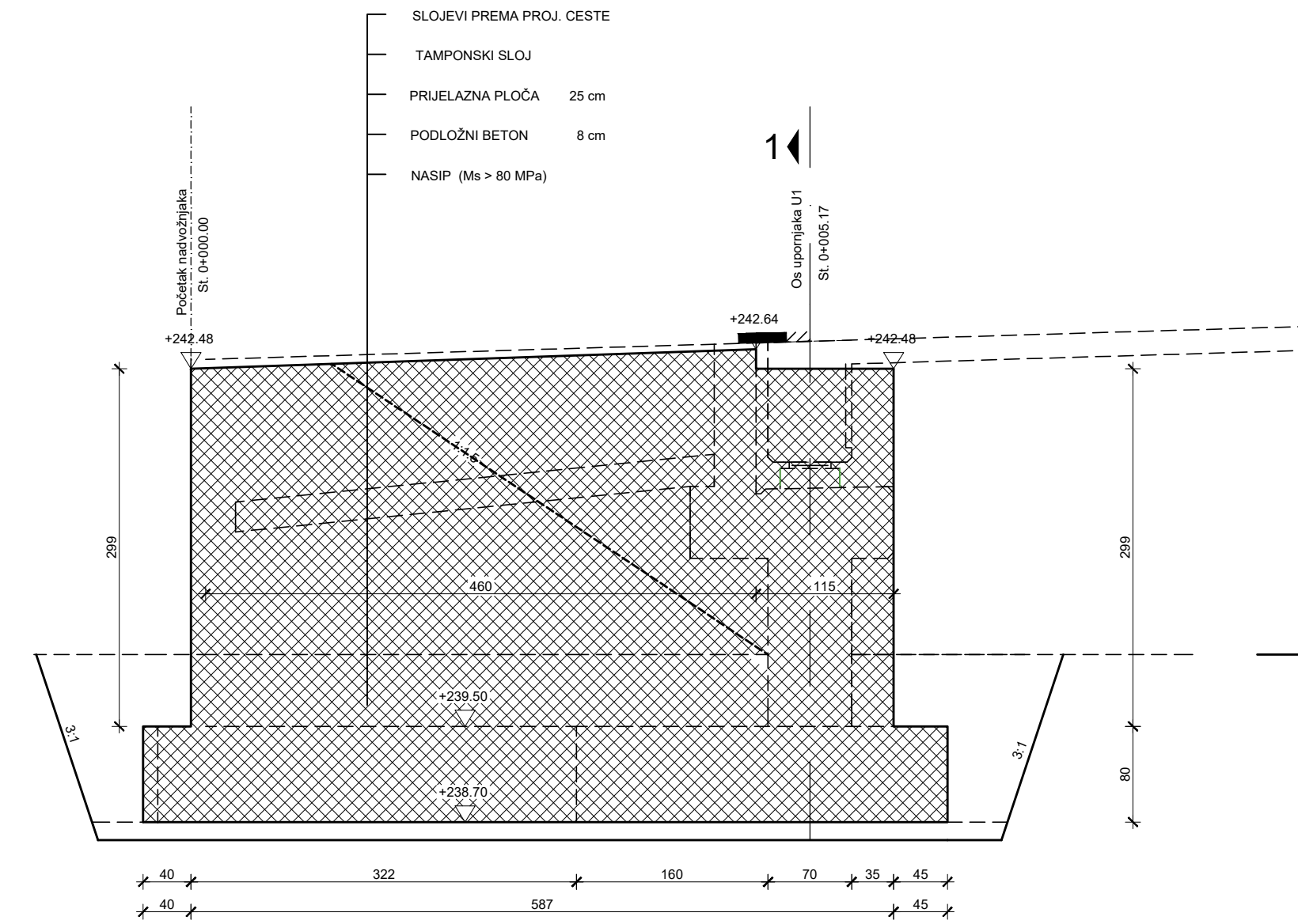
Presjek 6-6
