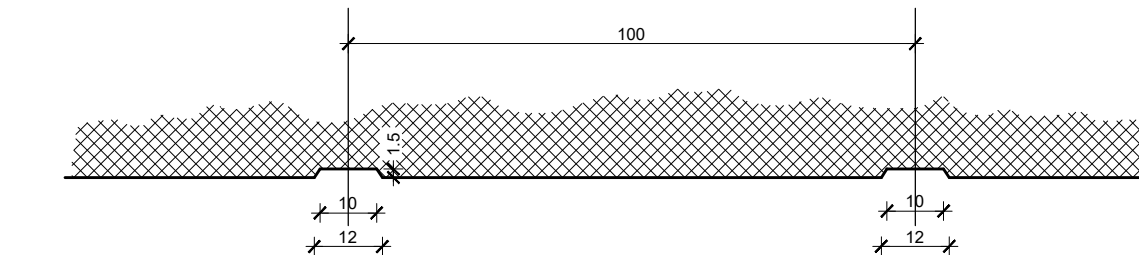
Detalj drenaže
