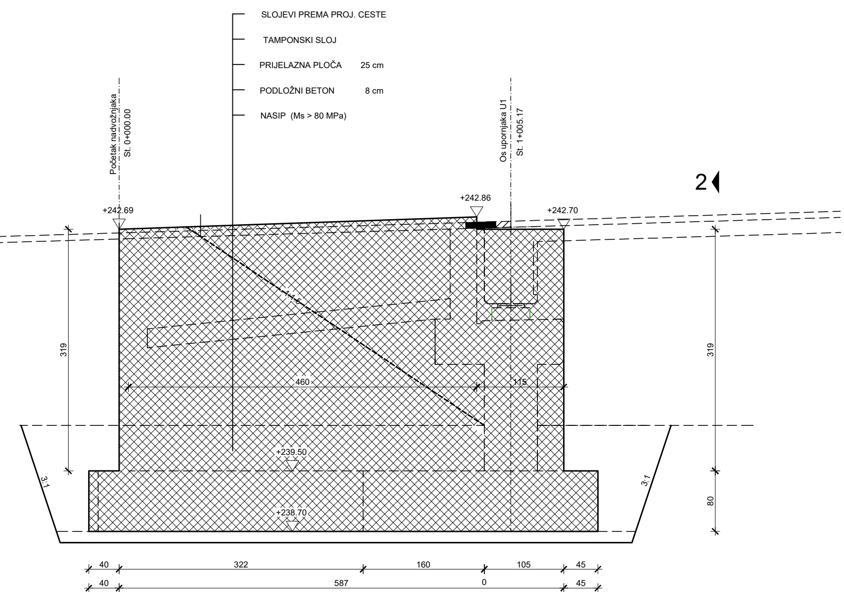
Presjek 5-5
