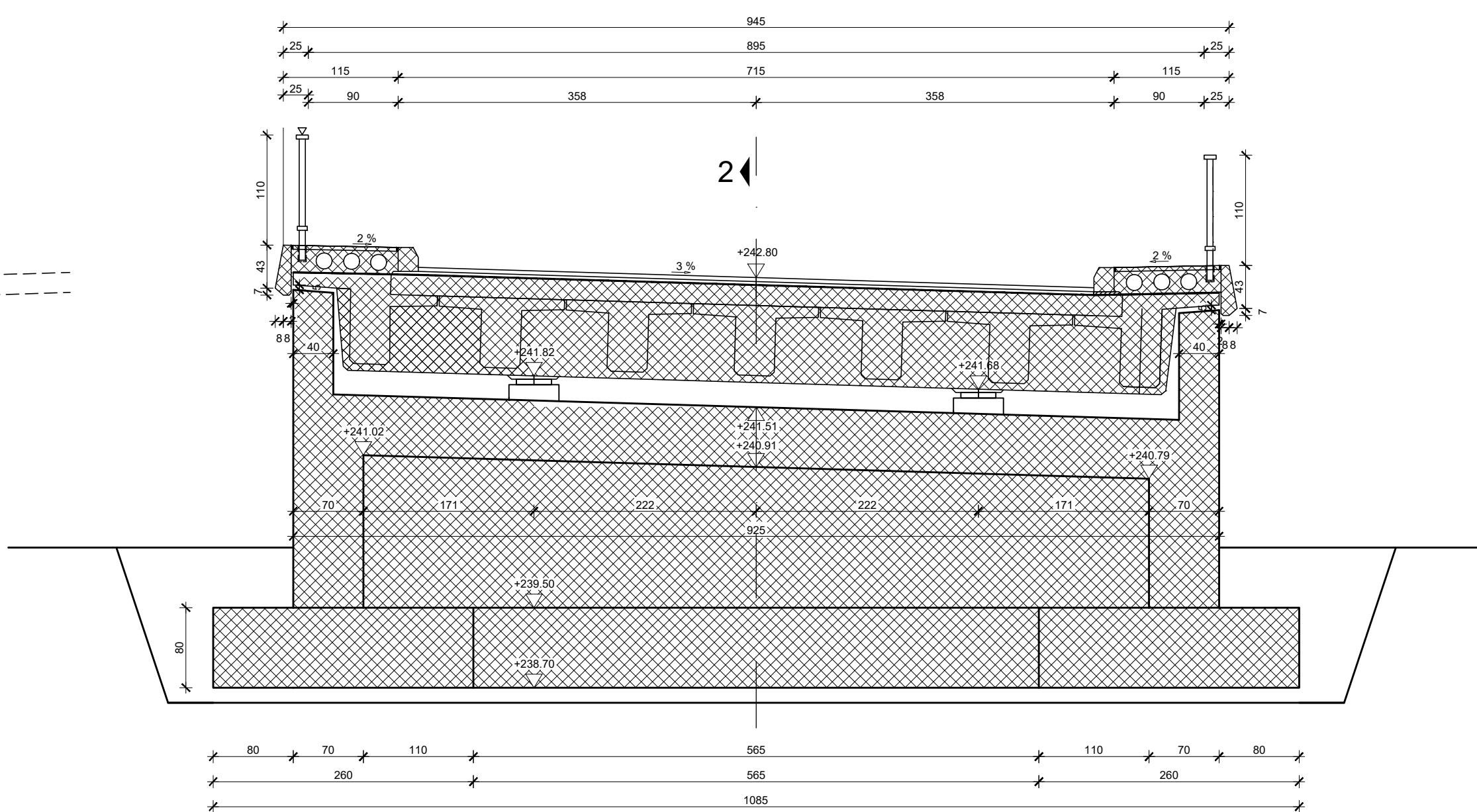
Presjek 1-1
