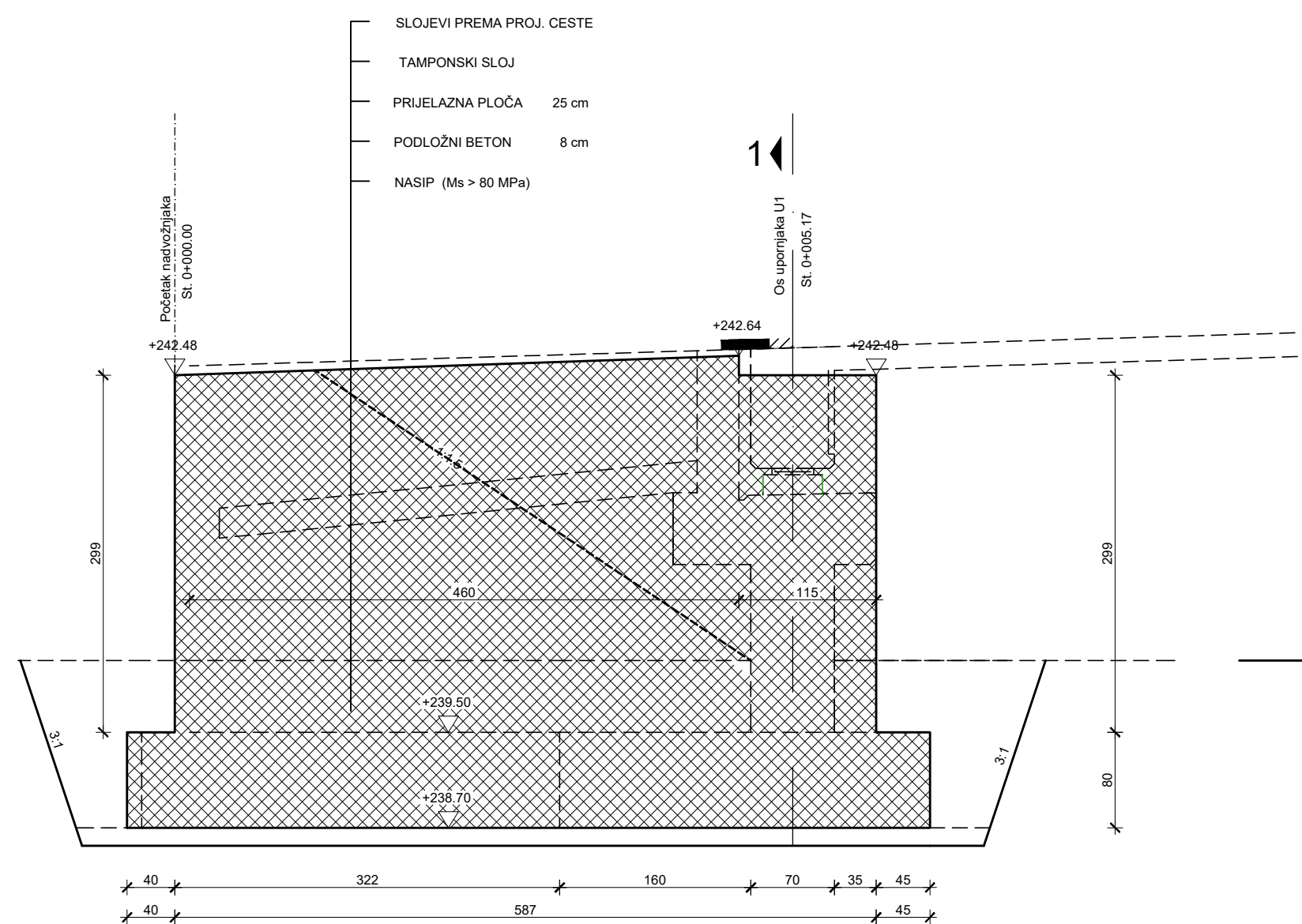
Presjek 6-6
