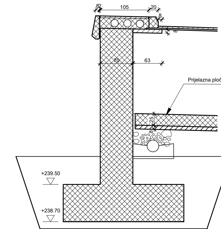
Presjek 7-7
