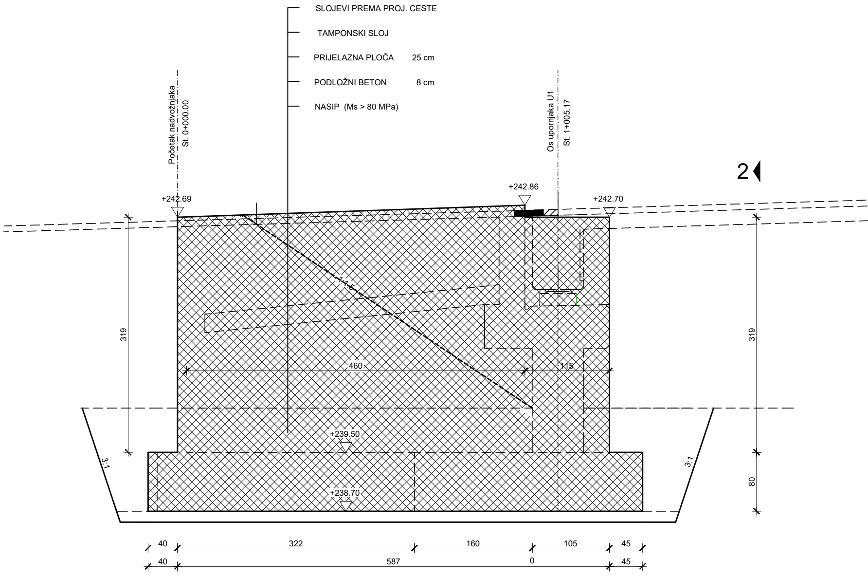
Presjek 5-5
