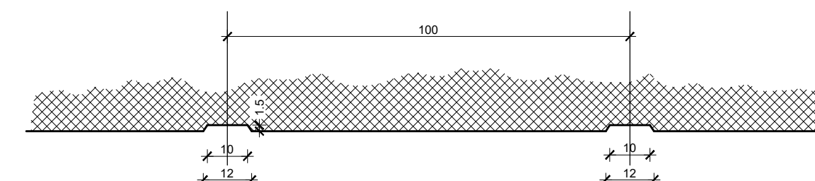
Detalj drenaže
