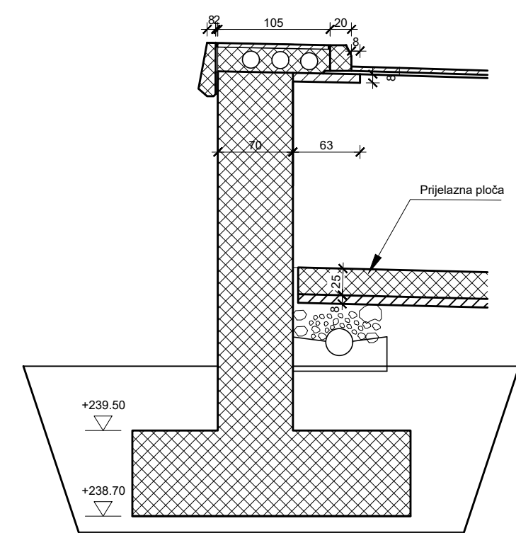
Presjek 7-7
