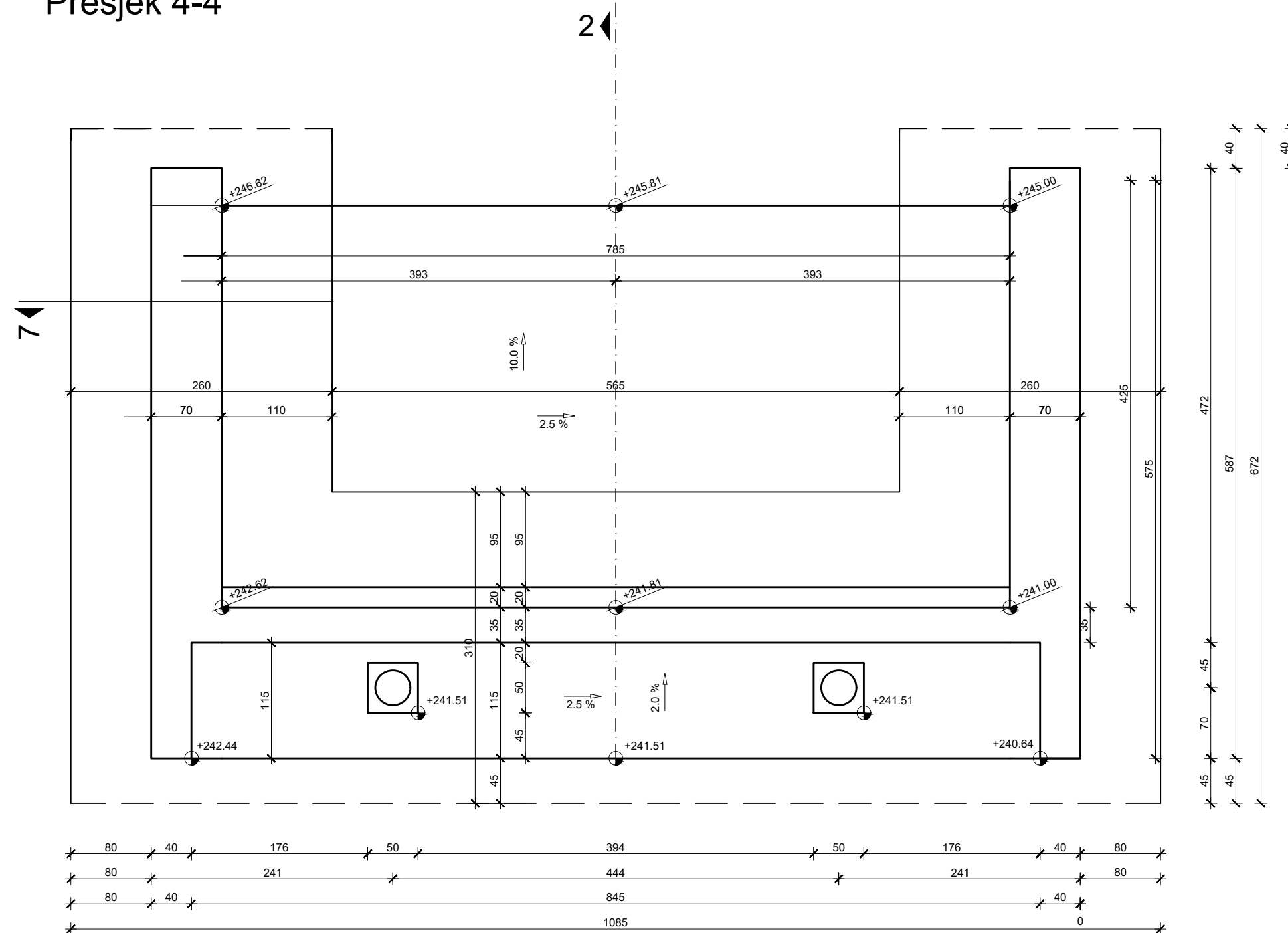
Presjek 4-4
