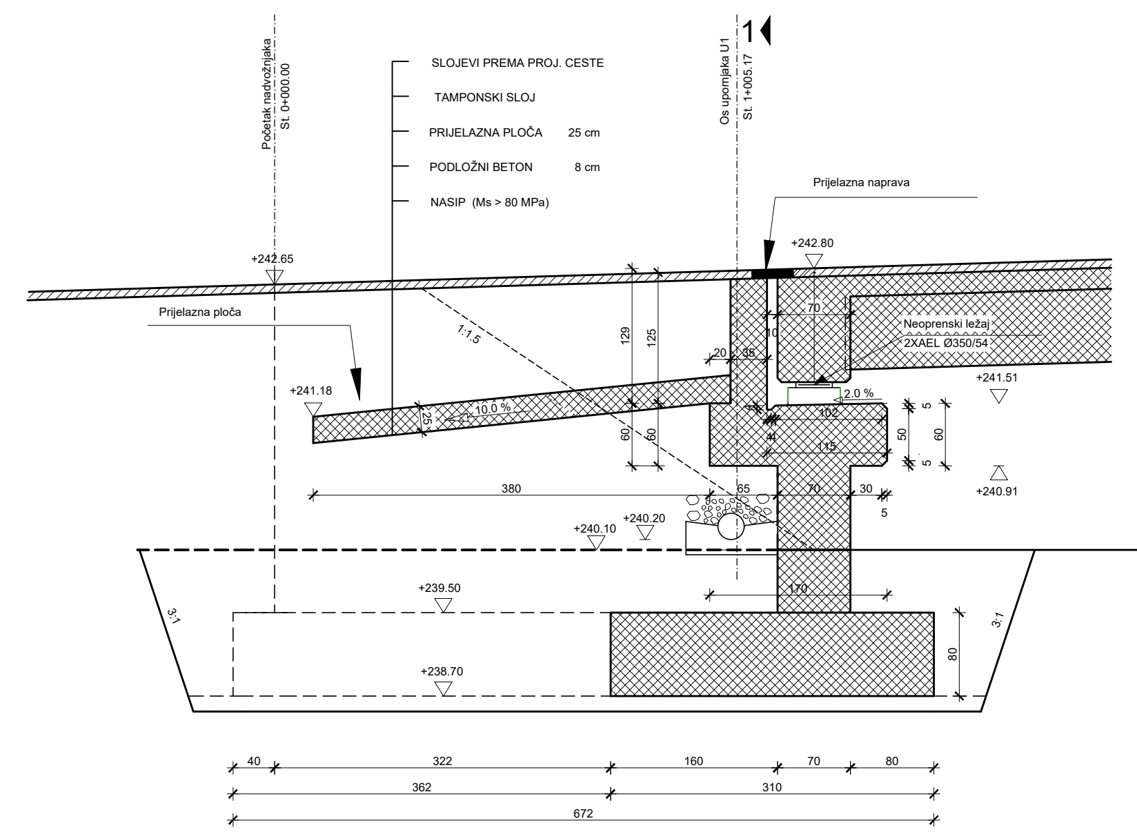
Presjek 3-3
