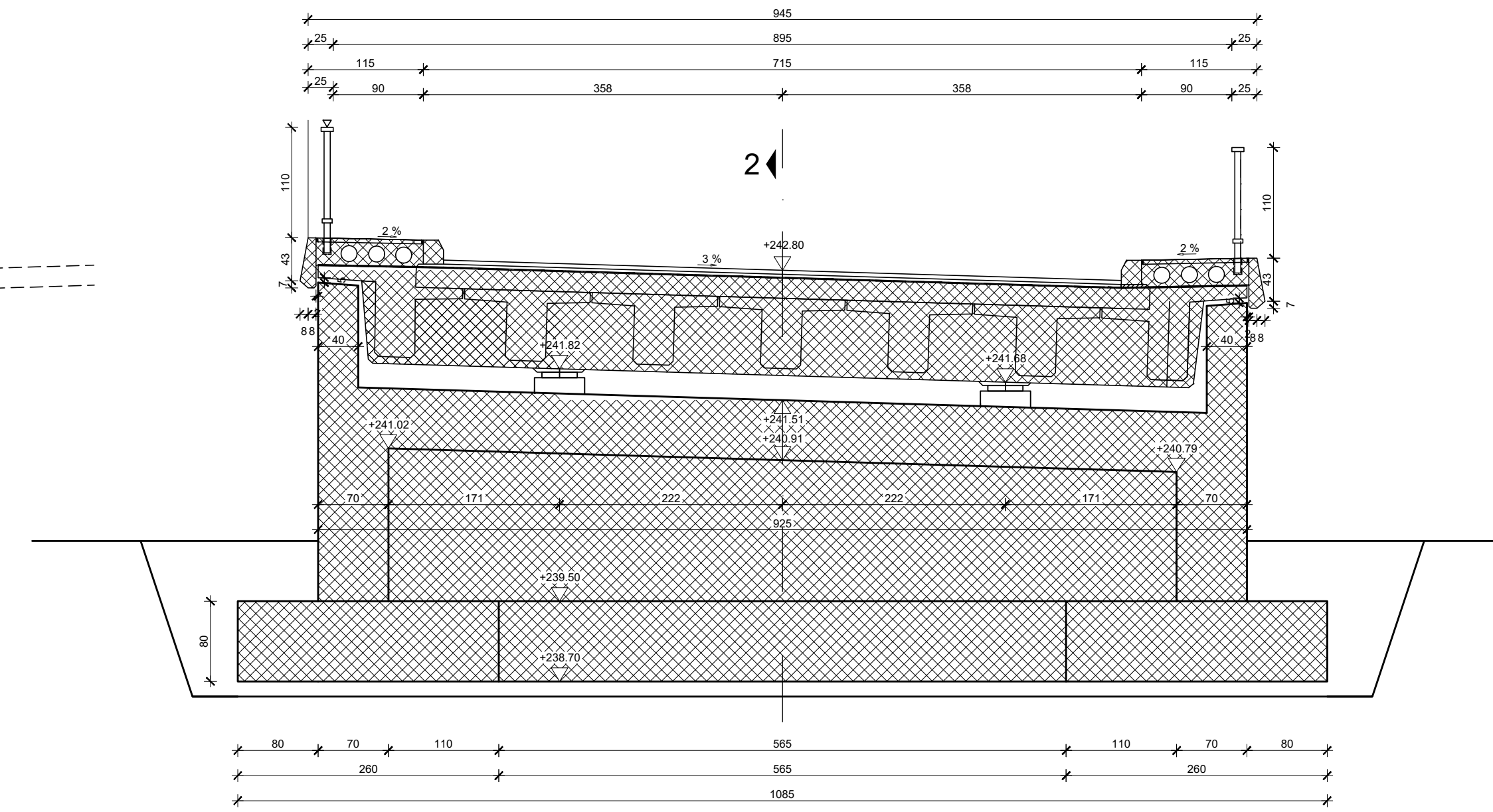
Presjek 1-1
