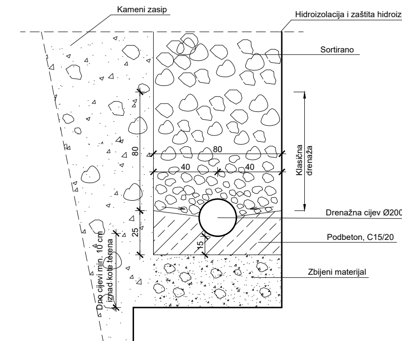
Detalj drenaže
