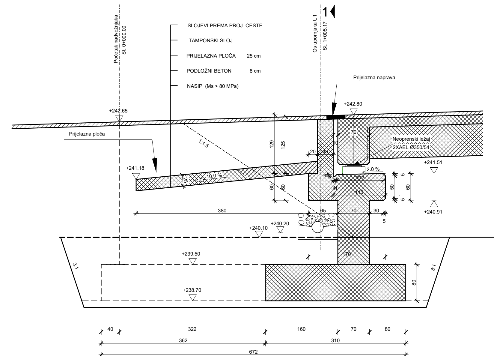
Presjek 3-3
