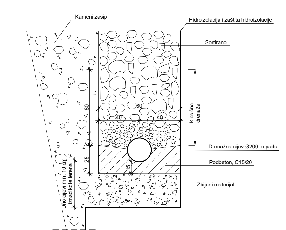
Detalj drenaze
