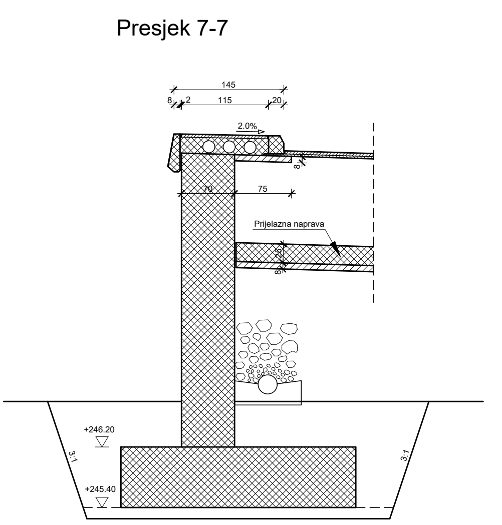
Presjek 7-7
