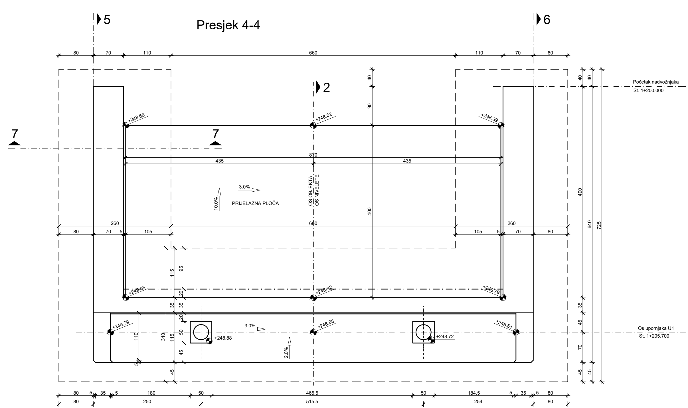
Presjek 4-4
