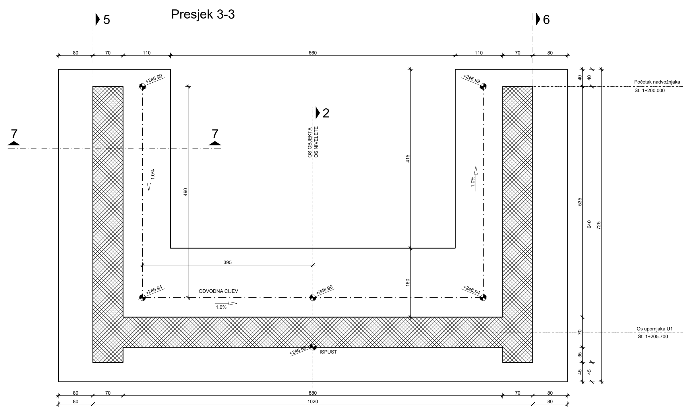
Presjek 3-3
