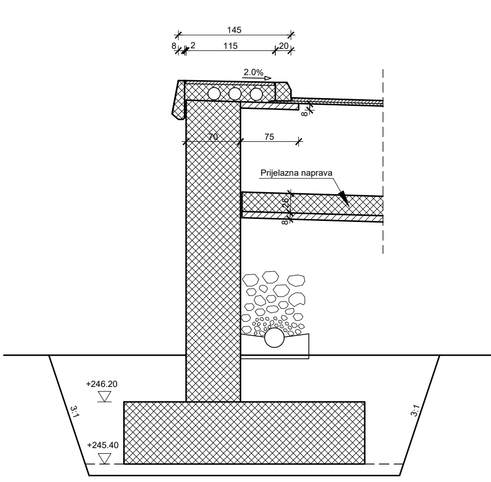
Presjek 7-7
