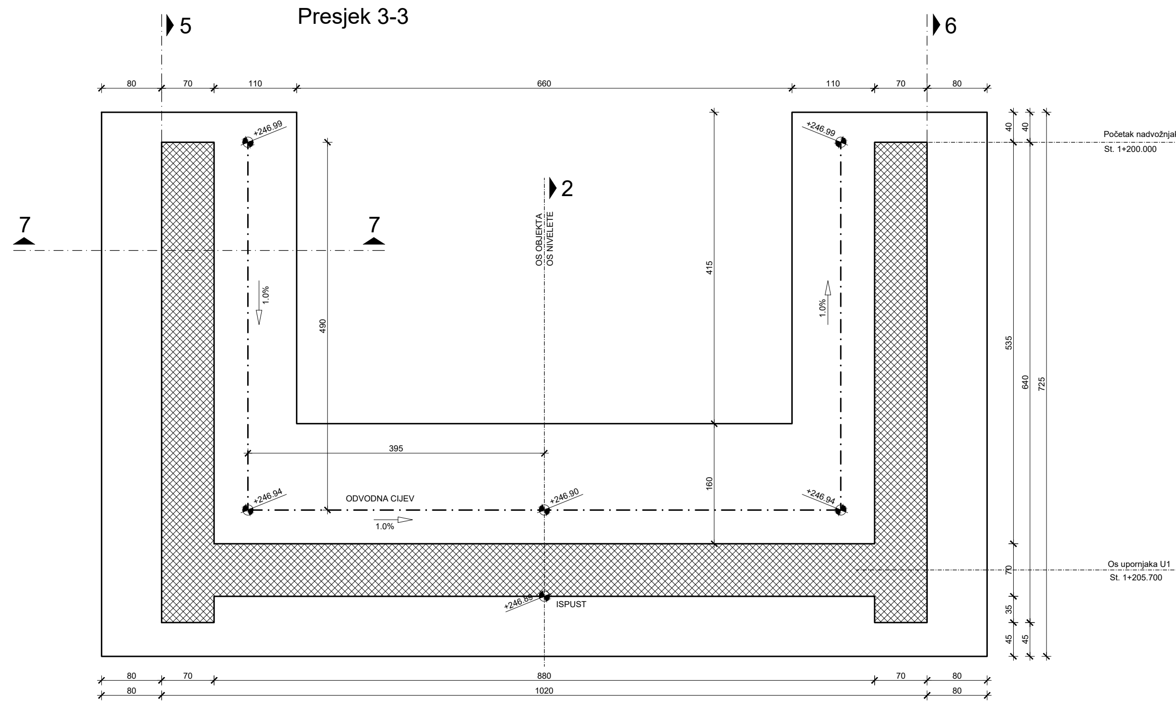
Presjek 3-3
