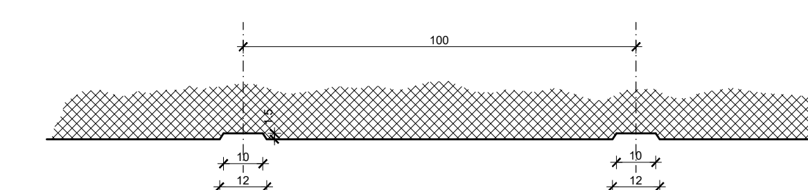
Detalj kanelura
