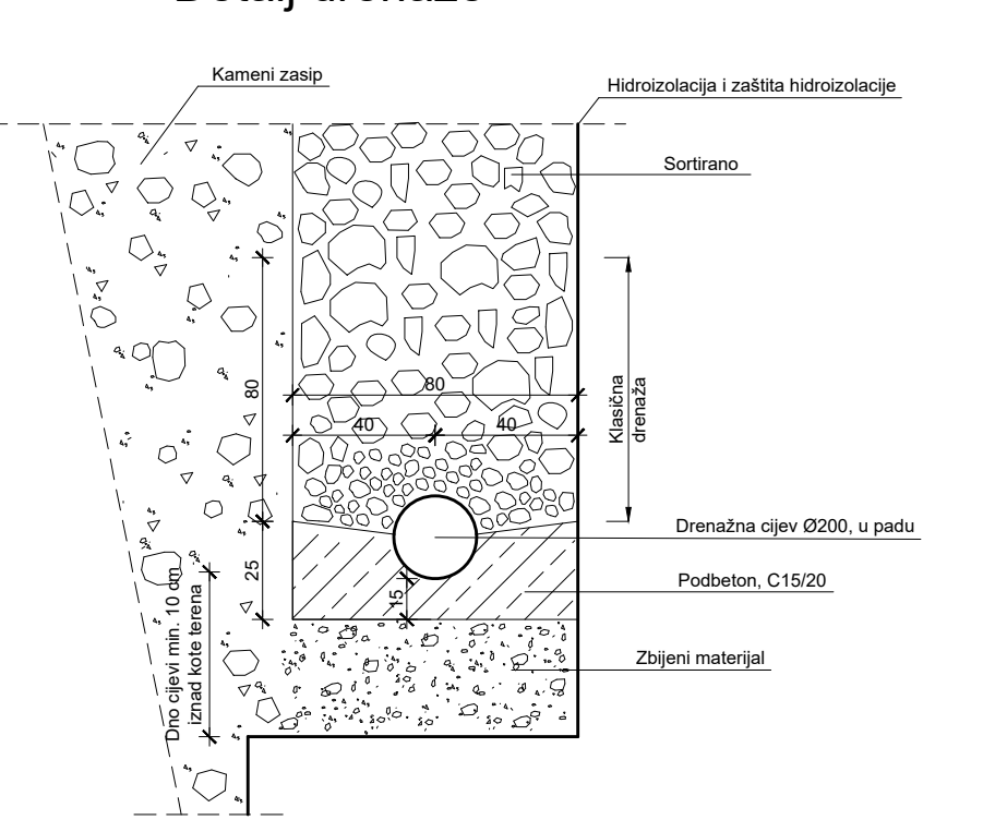
Detalj drenáže
