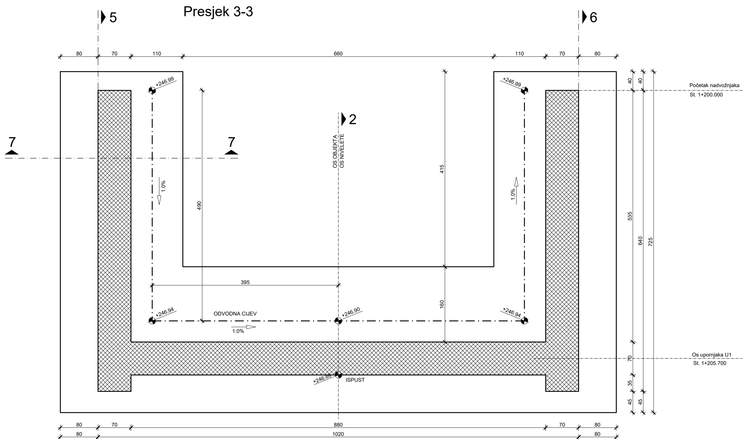
Presjek 3-3
