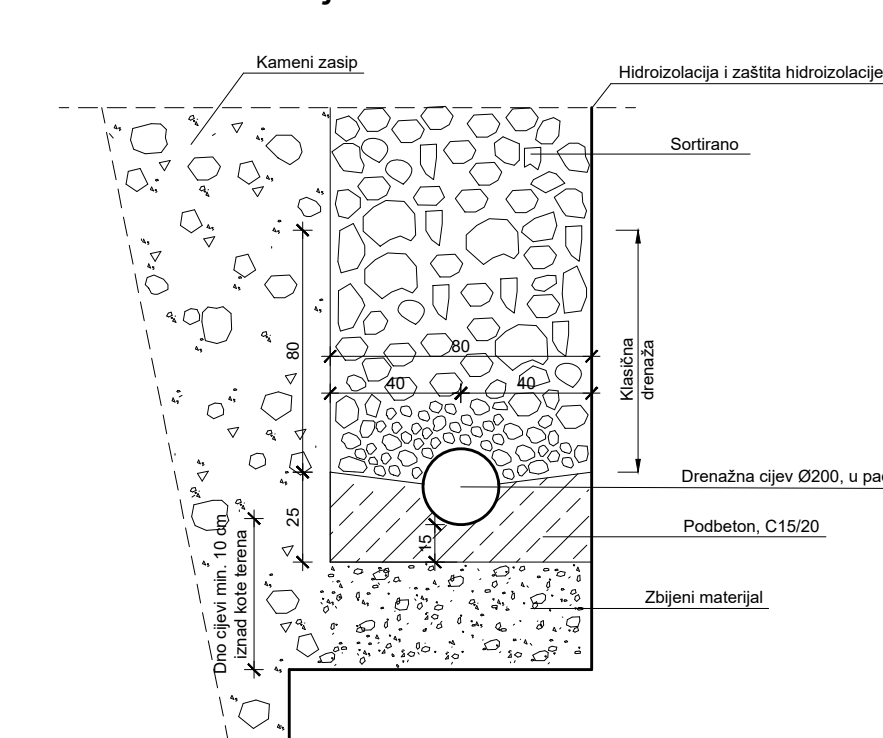
Detalj drenáže
