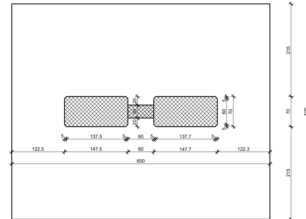
Presjek 4-4
