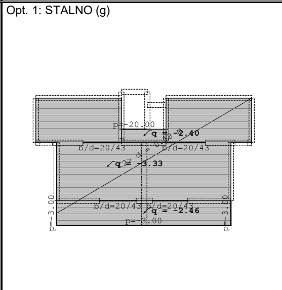
Nivo: PLOČA IZNAD 1.KATA POZ. 400 [8.85 m]
