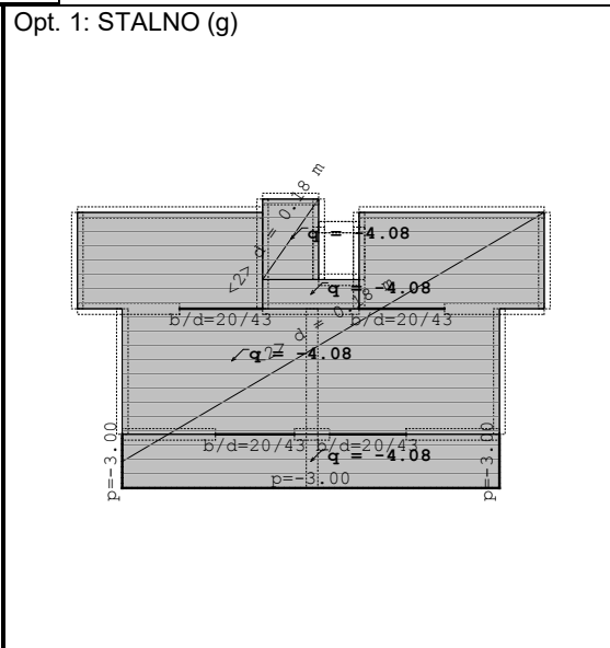
Nivo: PLOČA IZNAD 3.KATA POZ. 600 [14.75 m]
