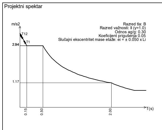
Slika 16. Proračun spektra ubrzanja tla za dane parametre
