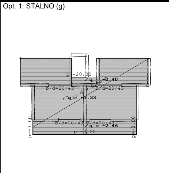
Nivo: PLOČA IZNAD 2.KATA POZ. 500 [11.80 m]
