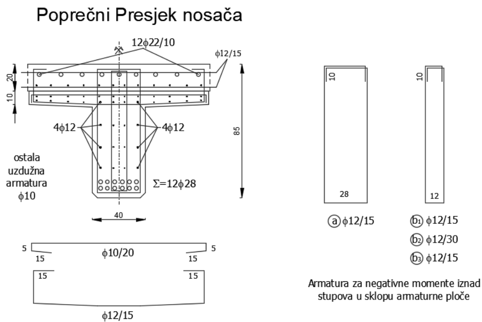
Slika 34. Prikaz armiranja nosača u presjeku
