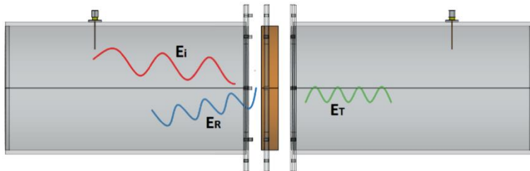
Slika 3. Eksperimentalna postavka
