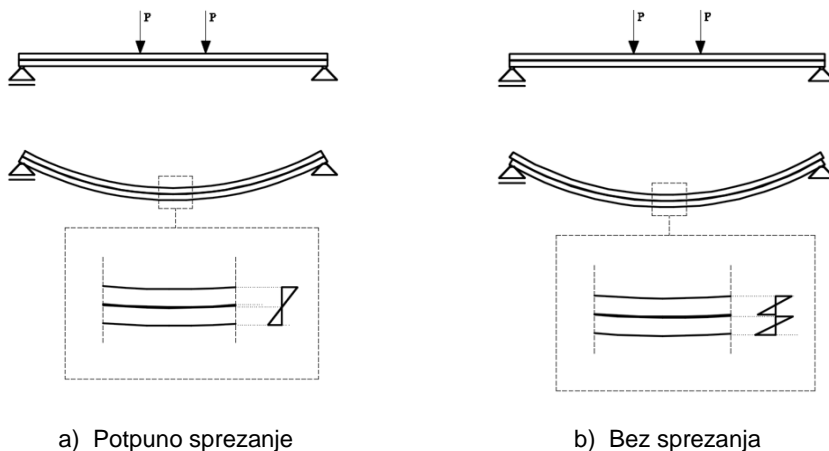
Slika 1. Prikaz raspodjele naprezanja na laminiranom nosaču za dva krajnja slučaja ponašanja međusloja – potpuno sprezanje i bez sprezanja [13]
