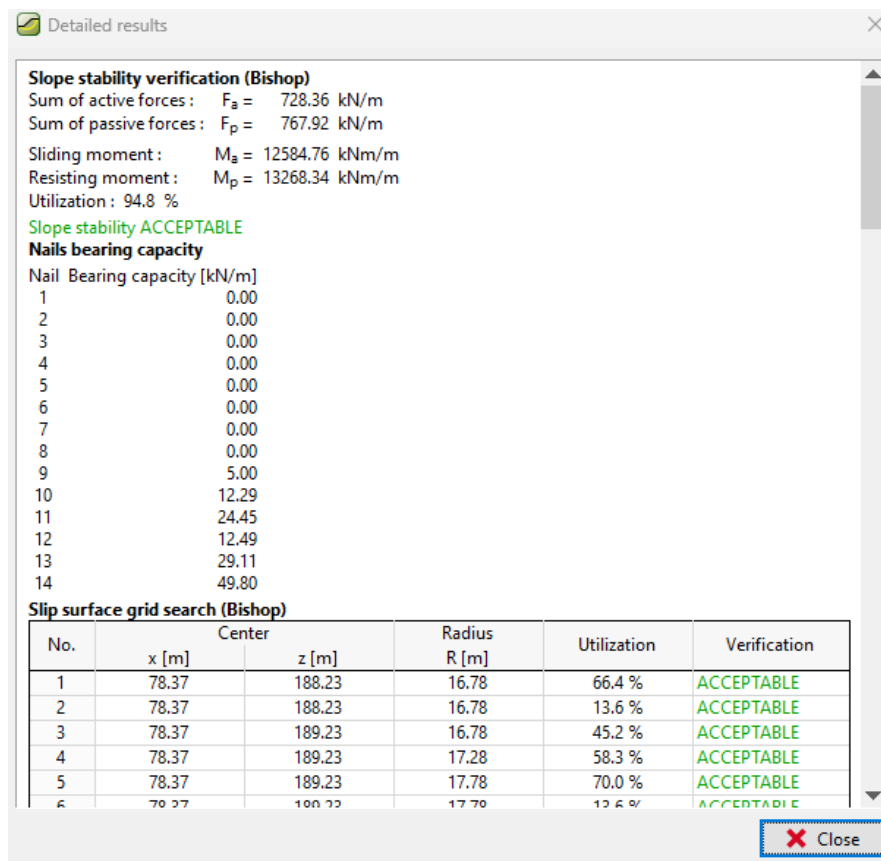
Slika 44. Nosivost štapnih sidara desne strane ulaznog predusjeka tunela
