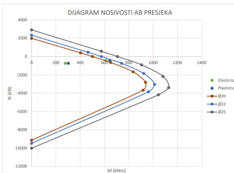
Slika 6.65. Dijagram interakcije (nosivosti) AB presjeka 60x60
