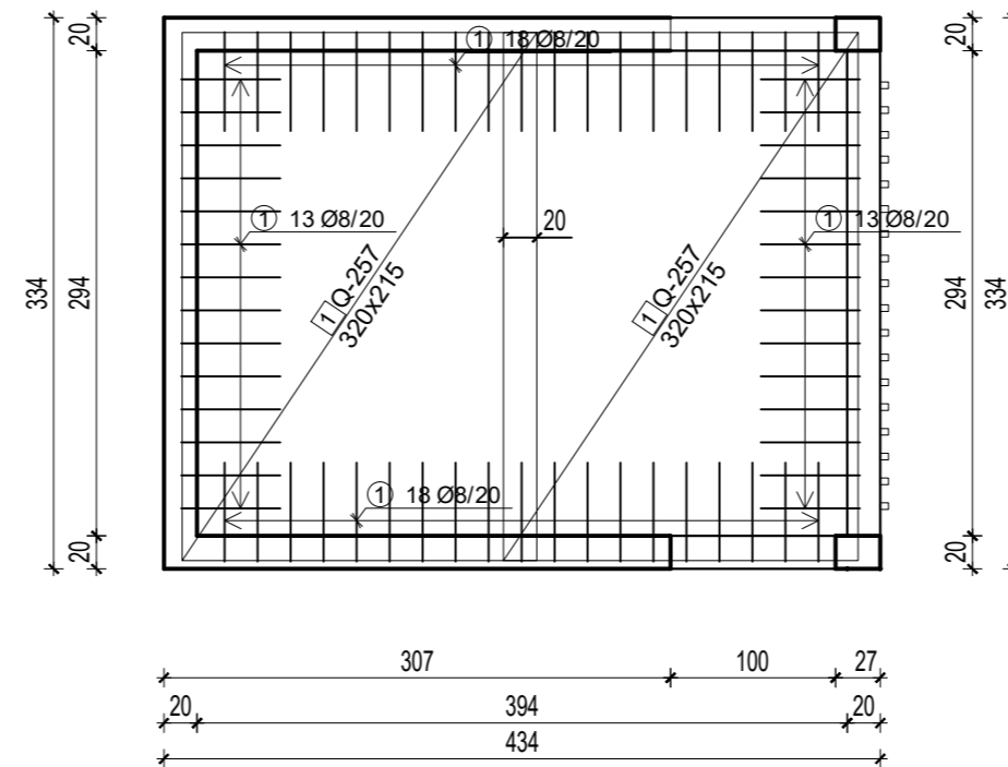
Mreže - specifikacija
