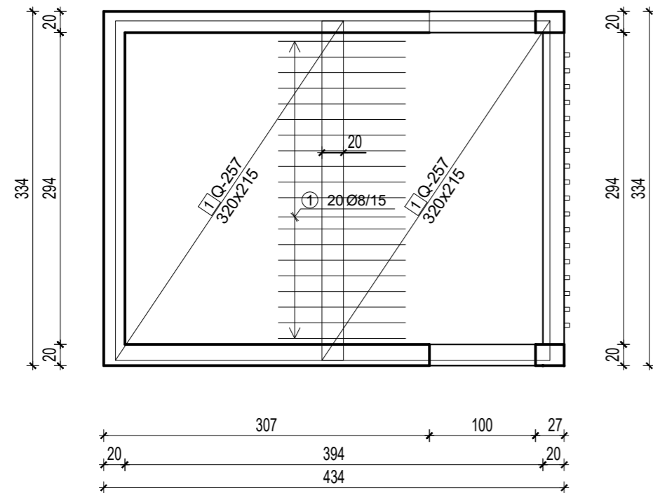
Mreže - specifikacija
