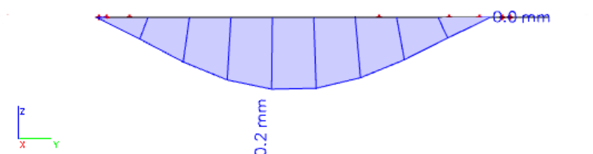
Slika 10.77 Dijagram progiba grede za GSU
