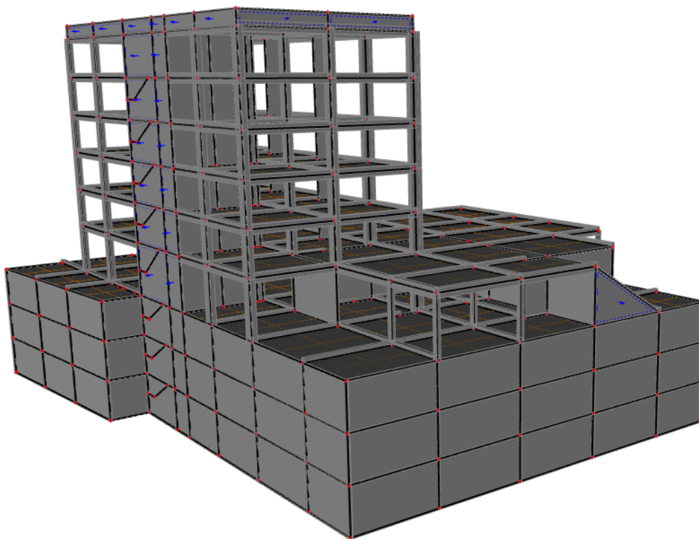
5.2 Renderirani prikaz modela zgrade - aksonometrija II
