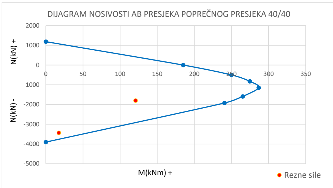
10.25 Dijagram nosivosti
