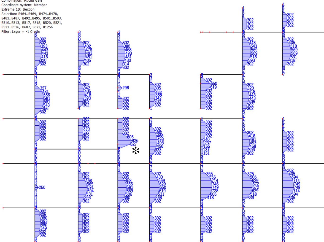
9.56 Površina potrebne armature - donja zona - Y smjer
