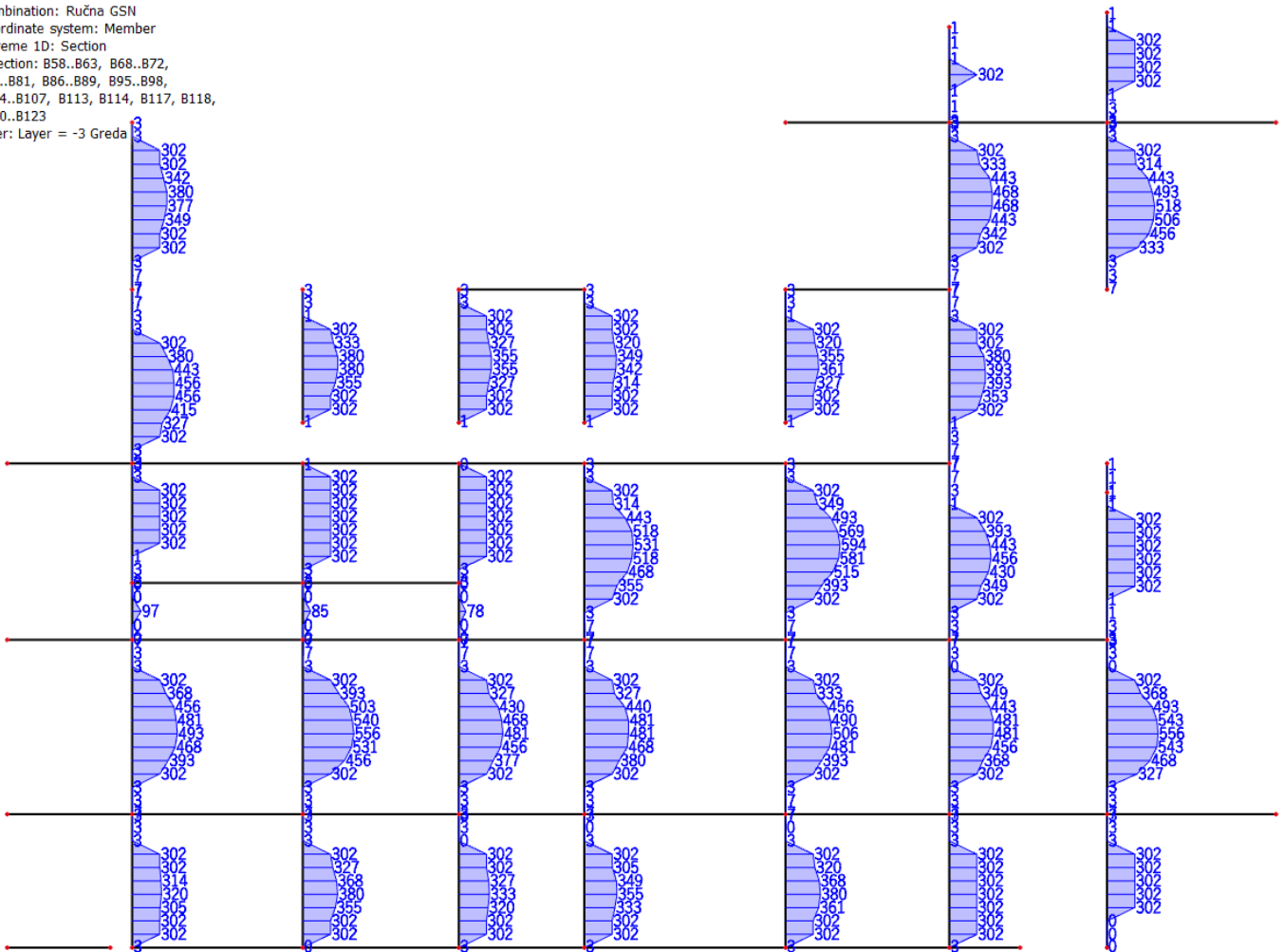
9.64 Površina potrebne armature - donja zona - Y smjer
