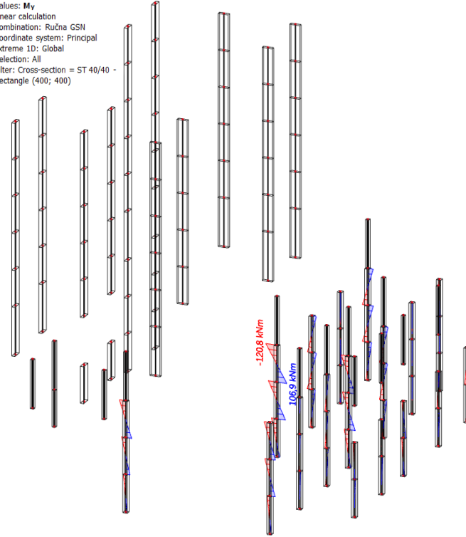
10.18 Prikaz momenta savijanja M_y
