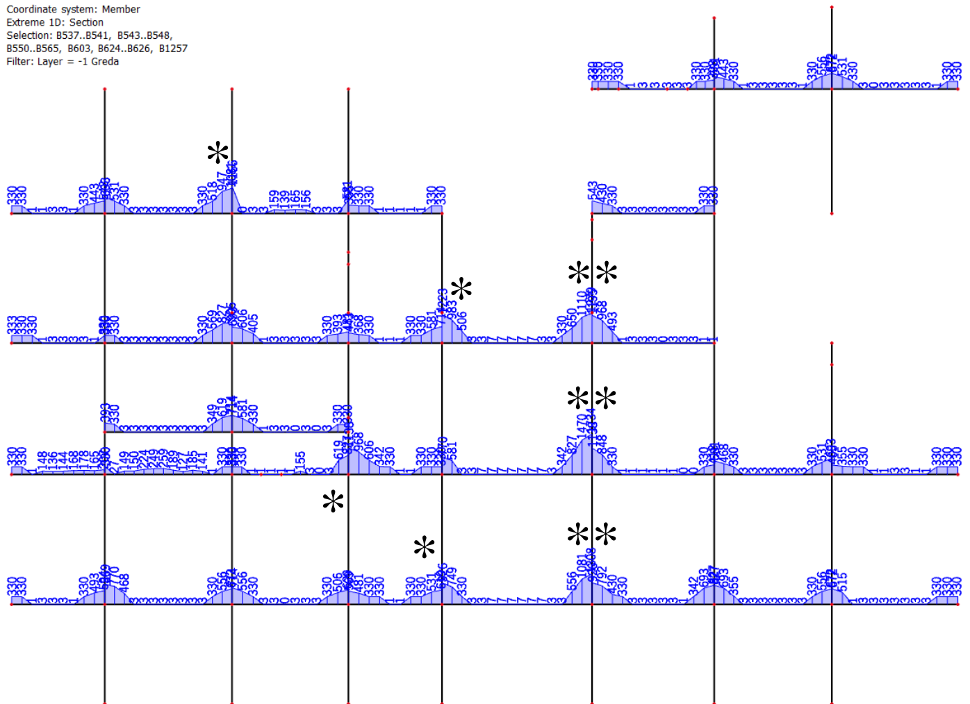
9.53 Površina potrebne armature - gornja zona - X smjer
