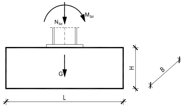
Slika 7.1. Prikaz temelja
