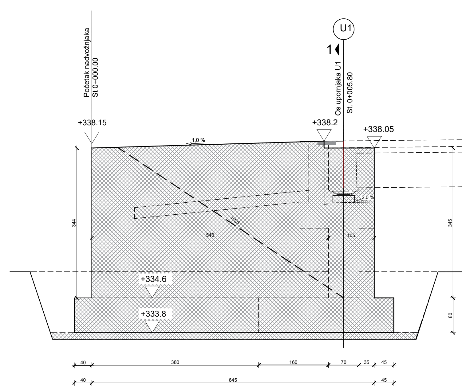
Presjek 5-5
