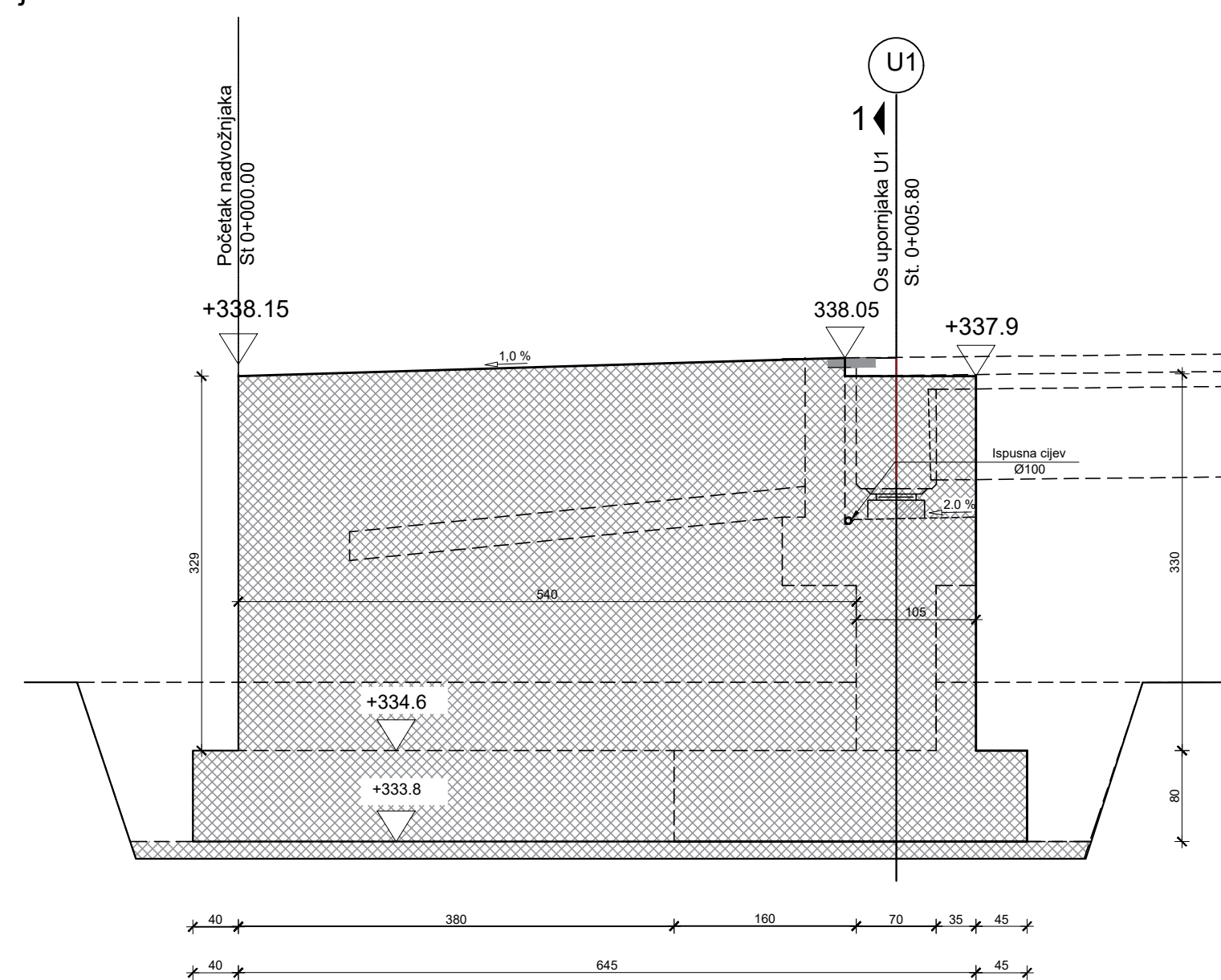
Presjek 6-6
