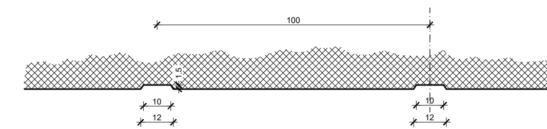
Detalj kanelura
