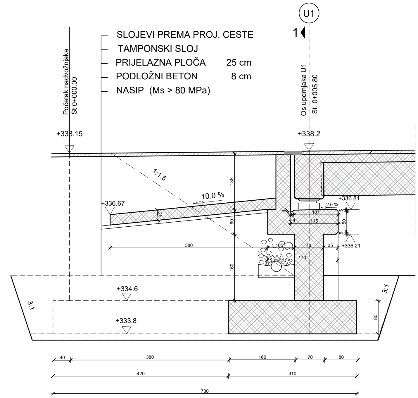
Presjek 4-4
