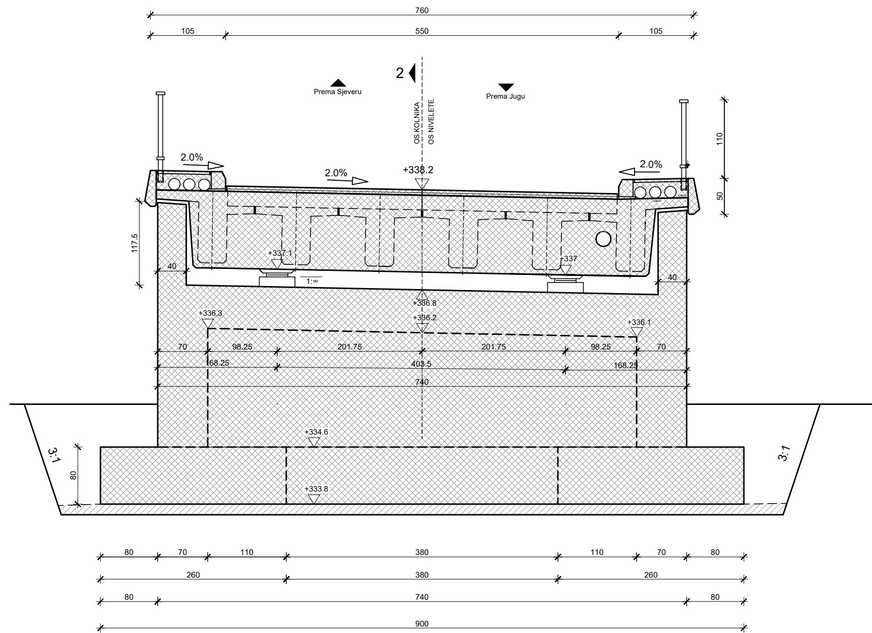
Presjek 6-6
