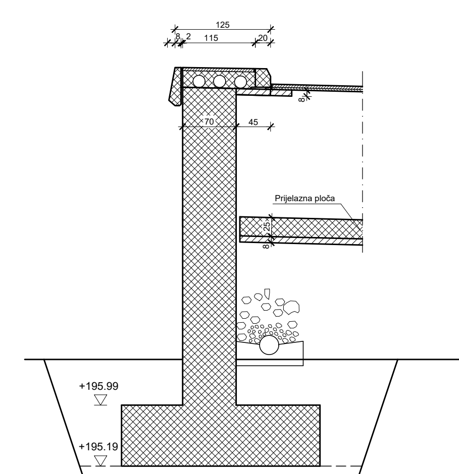
Presjek 7-7
