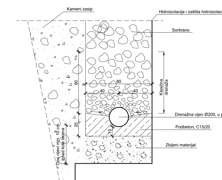
DETALJ DRENAŽE
