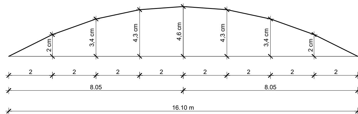
SHEMA NADVIŠENJA OPLATE NOSAČA
