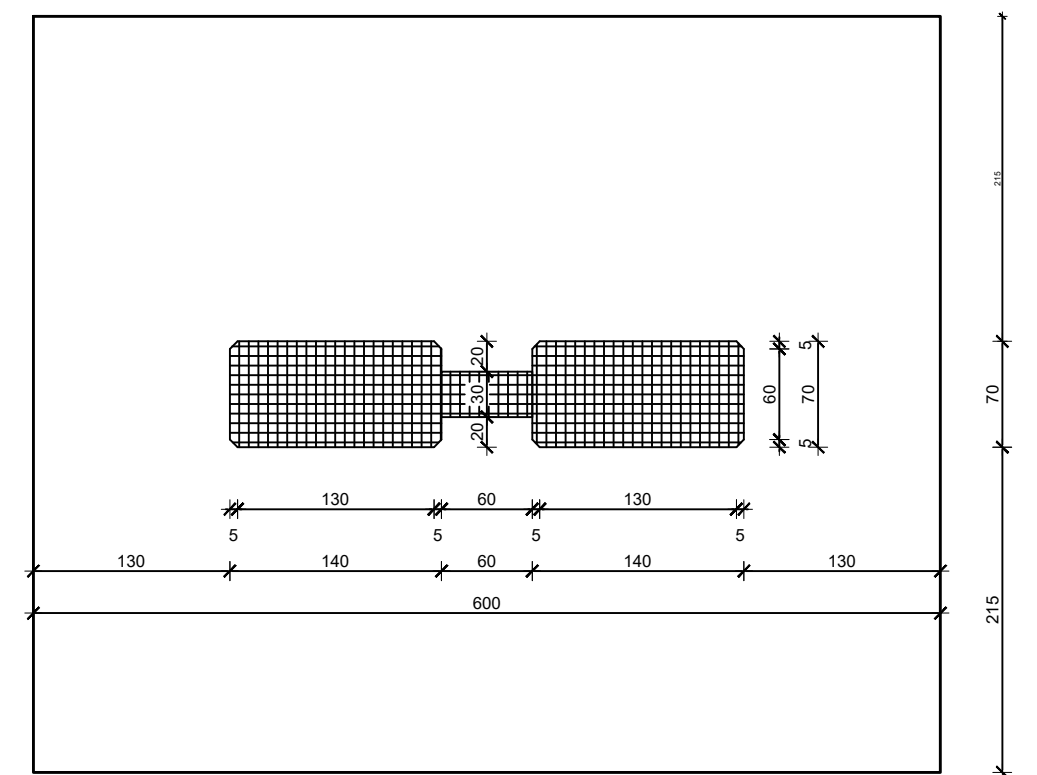
Presjek 4-4
