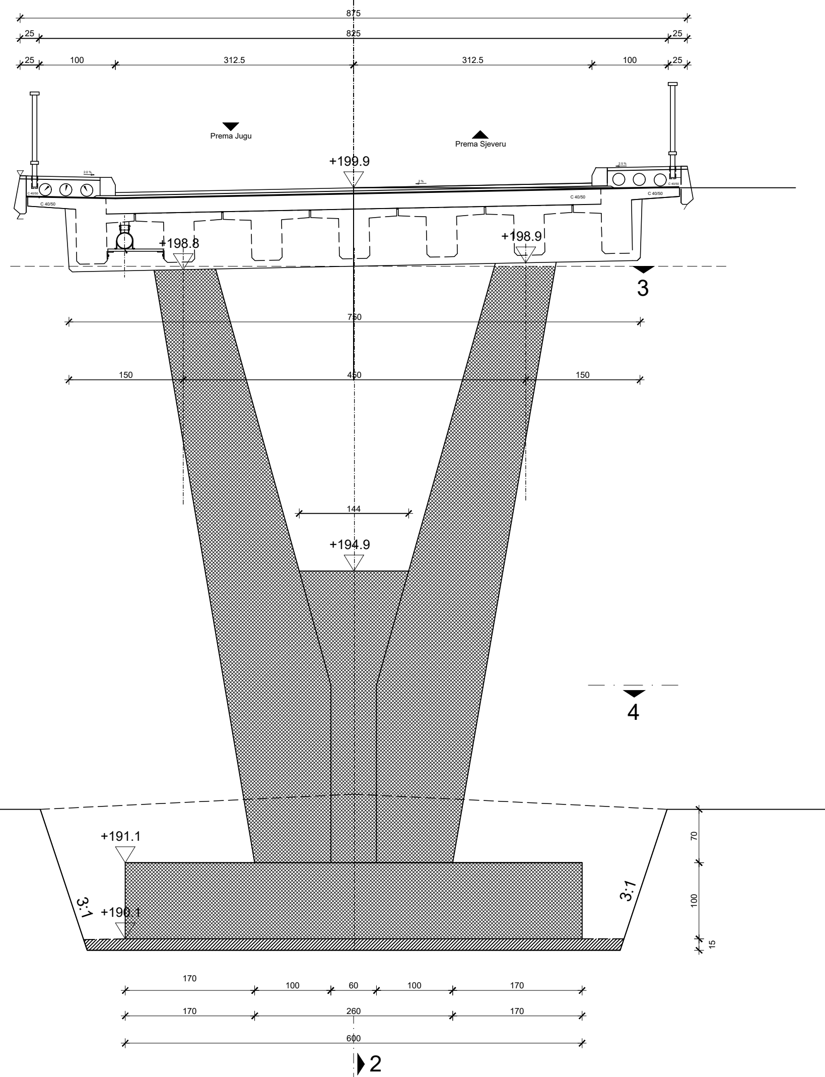
Presjek 1-1
