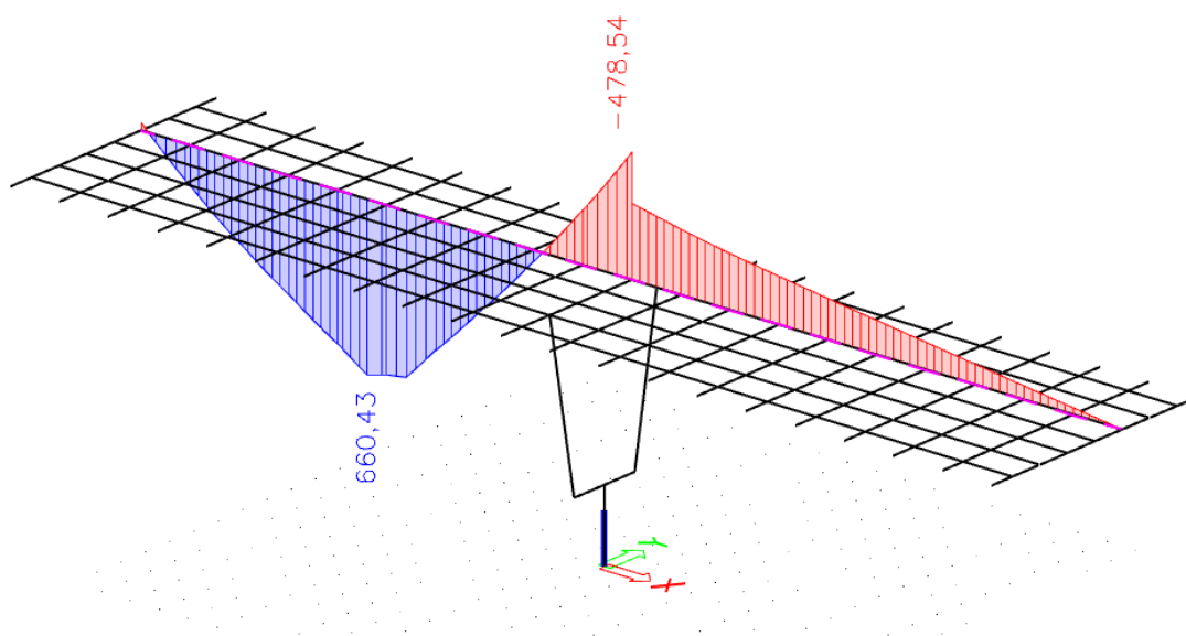
Slika 16. Pokretno – maksimalni moment u prvom polju – momenti ( M_y ) u kNm
