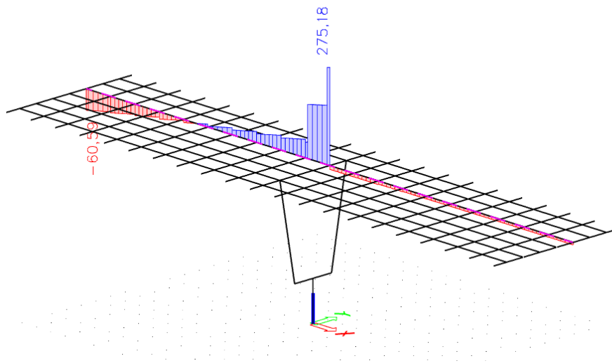
Slika 25. Pokretno – maksimalna poprečna sila pri stupu – poprečne sile ( V_z ) u kN
