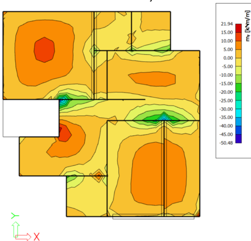
Moment m_y
