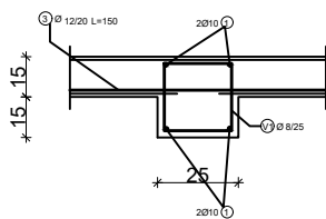
HORIZONTALAN SERKLAŽ 1:25
