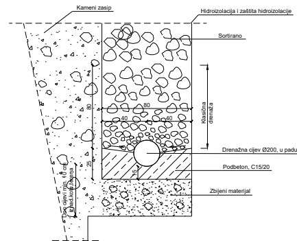
Detalj drenaze
