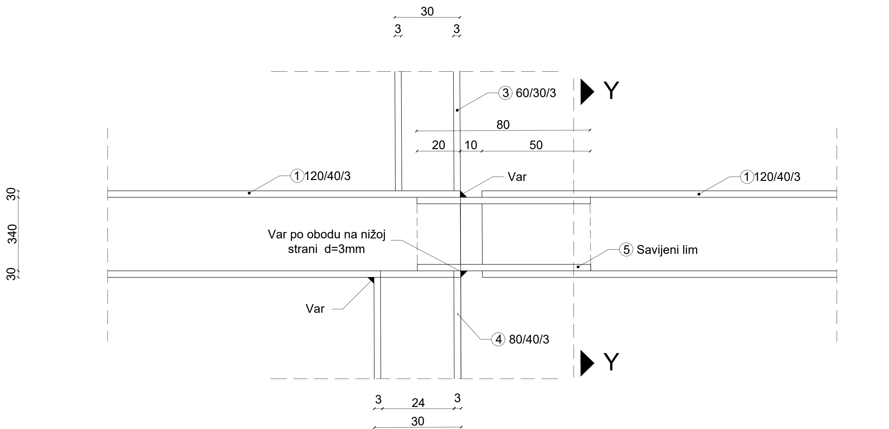
Detalj D 2 1:2
