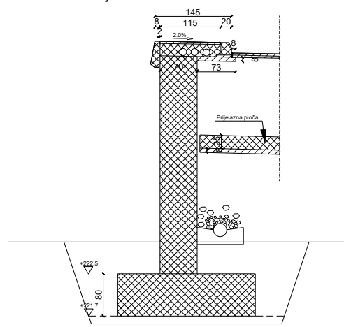
Presjek 7-7
