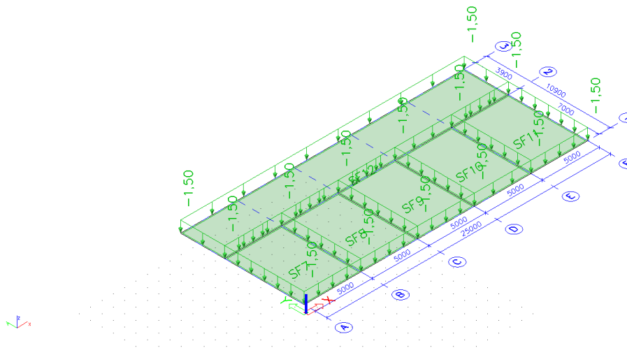
Slika 10.3: Pokretno opterećenje
