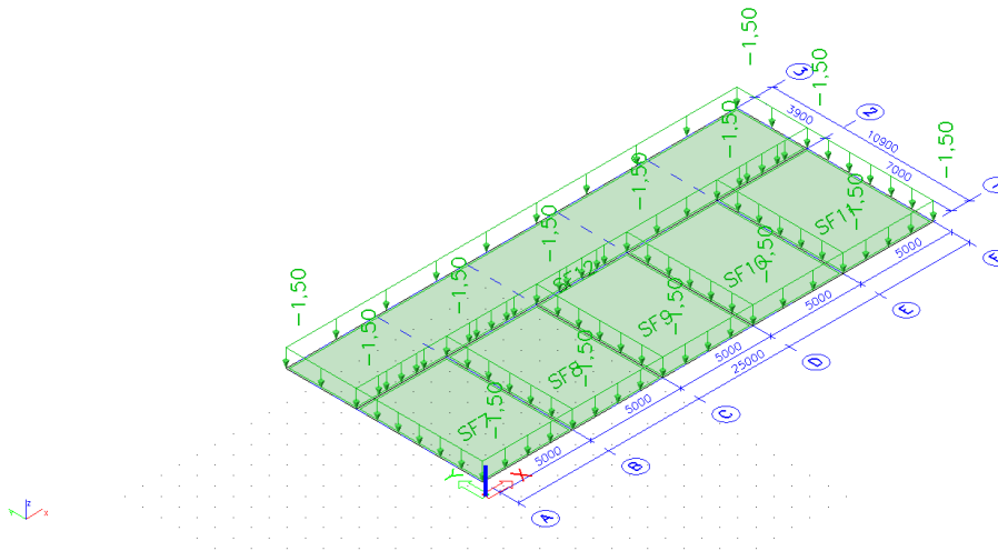
Slika 10.3: Pokretno opterećenje
