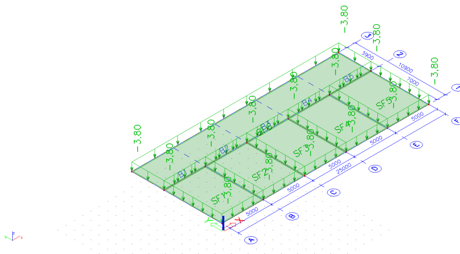
Slika 10.2: Stalno opterećenje
