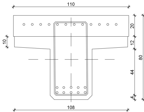
Slika 36. Dimenzije nosača
