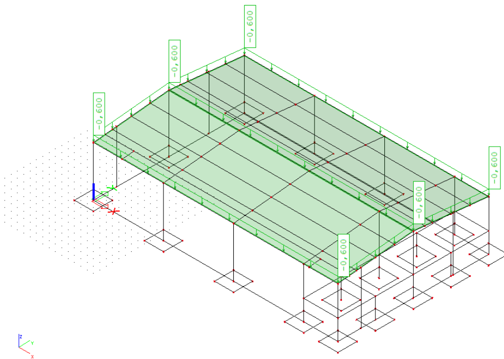
Slika 7.9 Dodatno stalno opterećenja na krovu
