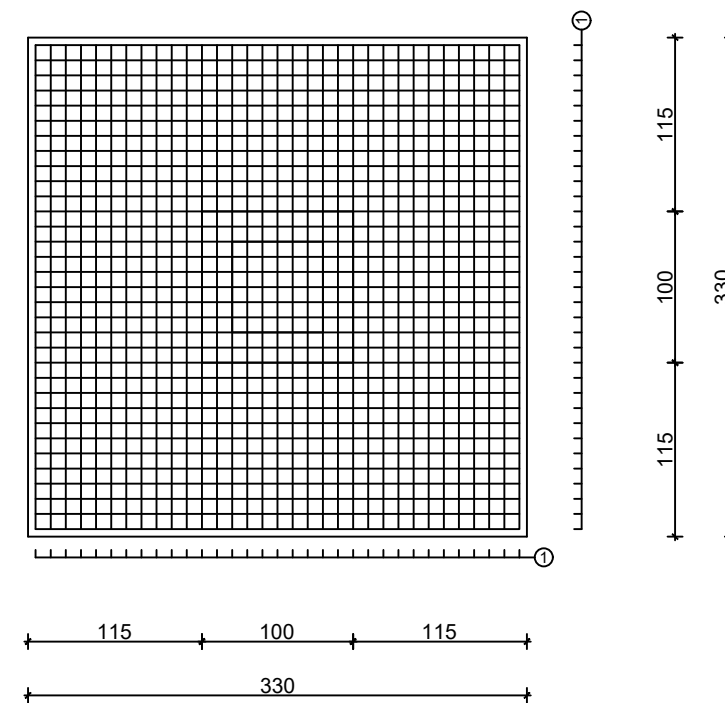
PRESJEK 4-4
