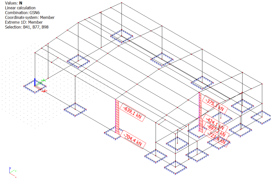
Slika 9.17 Prikaz uzdužne sile za odabrane stupove S10 i S2 za GSN6
