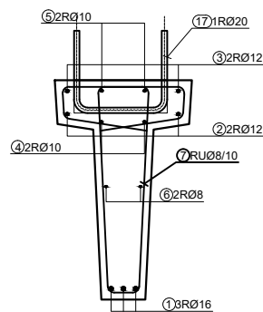
PRESJEK 2-2
