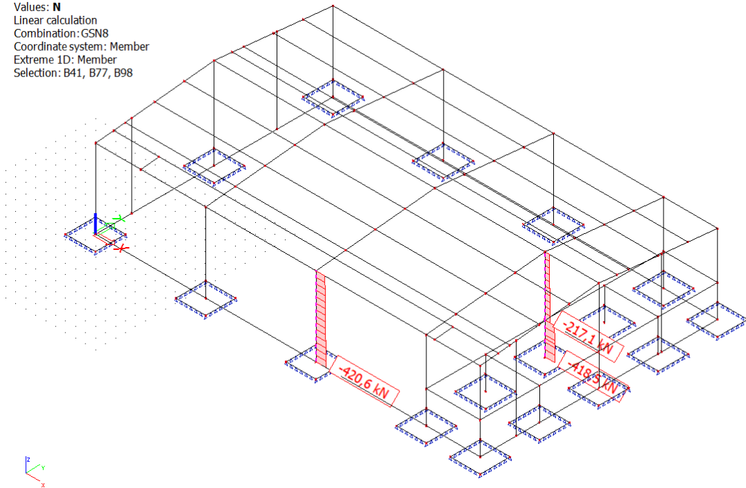
Slika 9.21 Prikaz uzdužne sile za odabrane stupove S10 i S2 za GSN8
