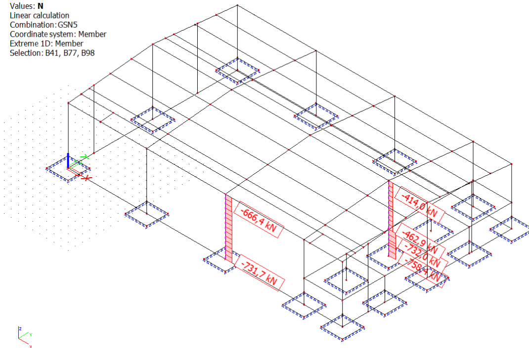
Slika 9.15 Prikaz uzdužne sile za odabrane stupove S10 i S2 za GSN5
