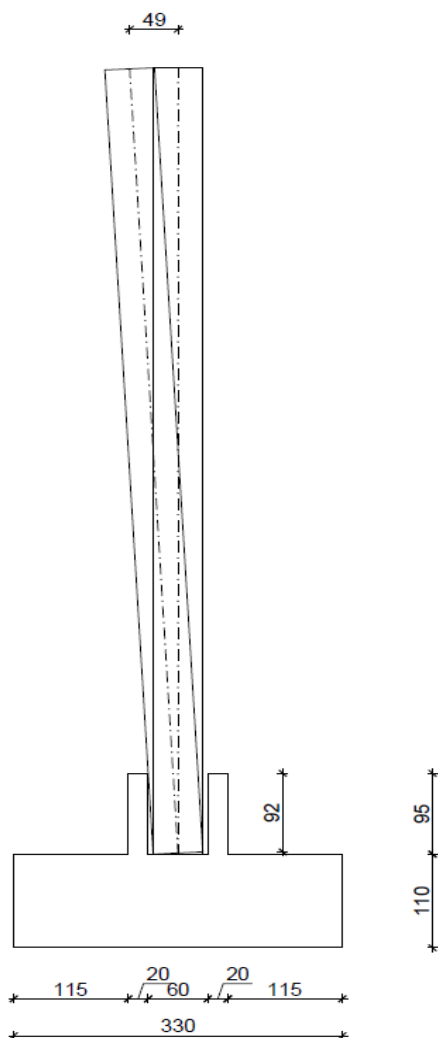
Slika 9.28 Ekscentricitet temelja
