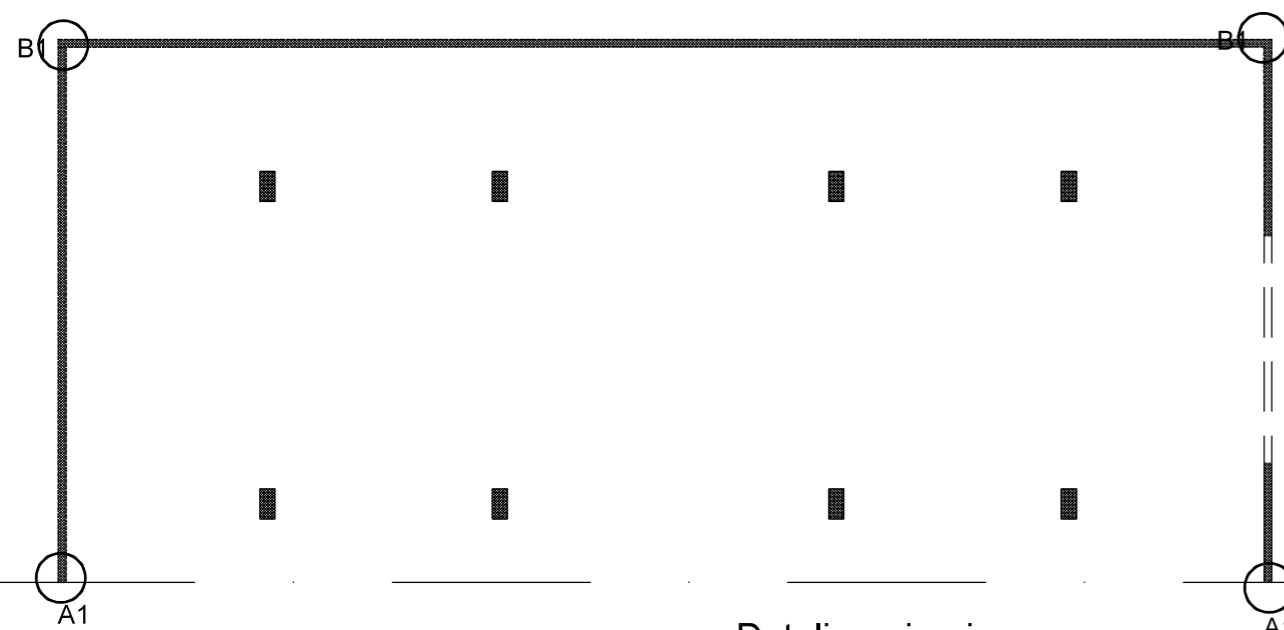
Detalj armiranja visokostijenog nosača
