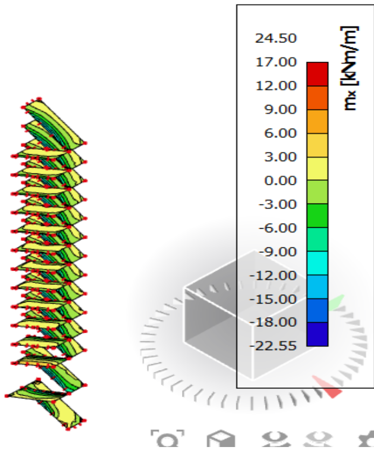
Slika 9.2. Moment savijanje globalni smjer X
