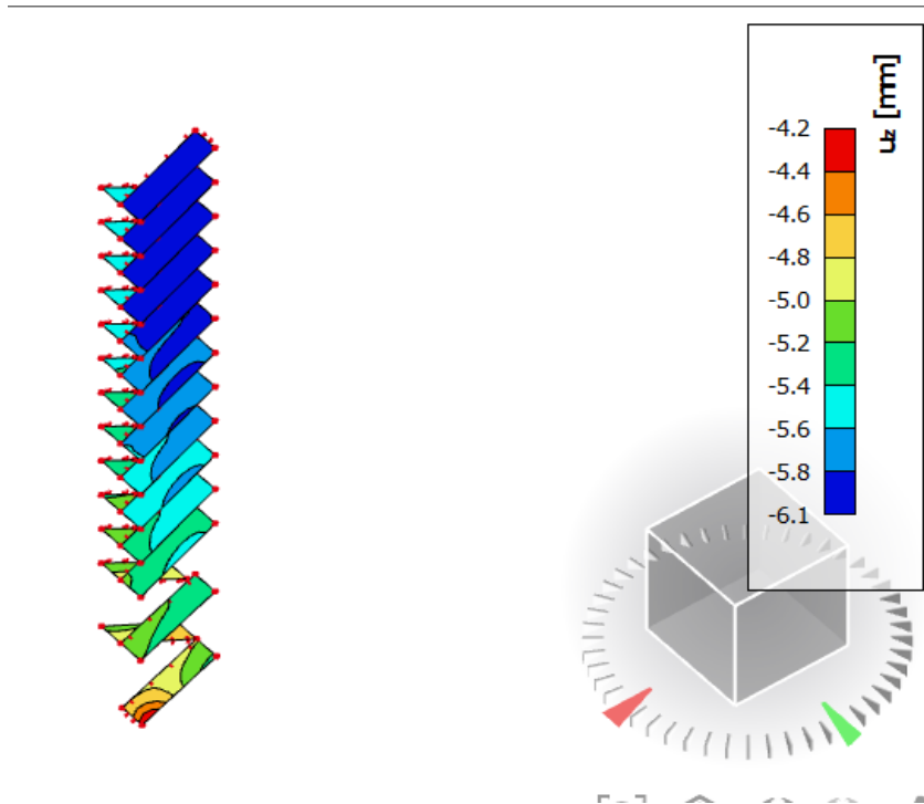
Slika 9.4. Progibi (mm)
