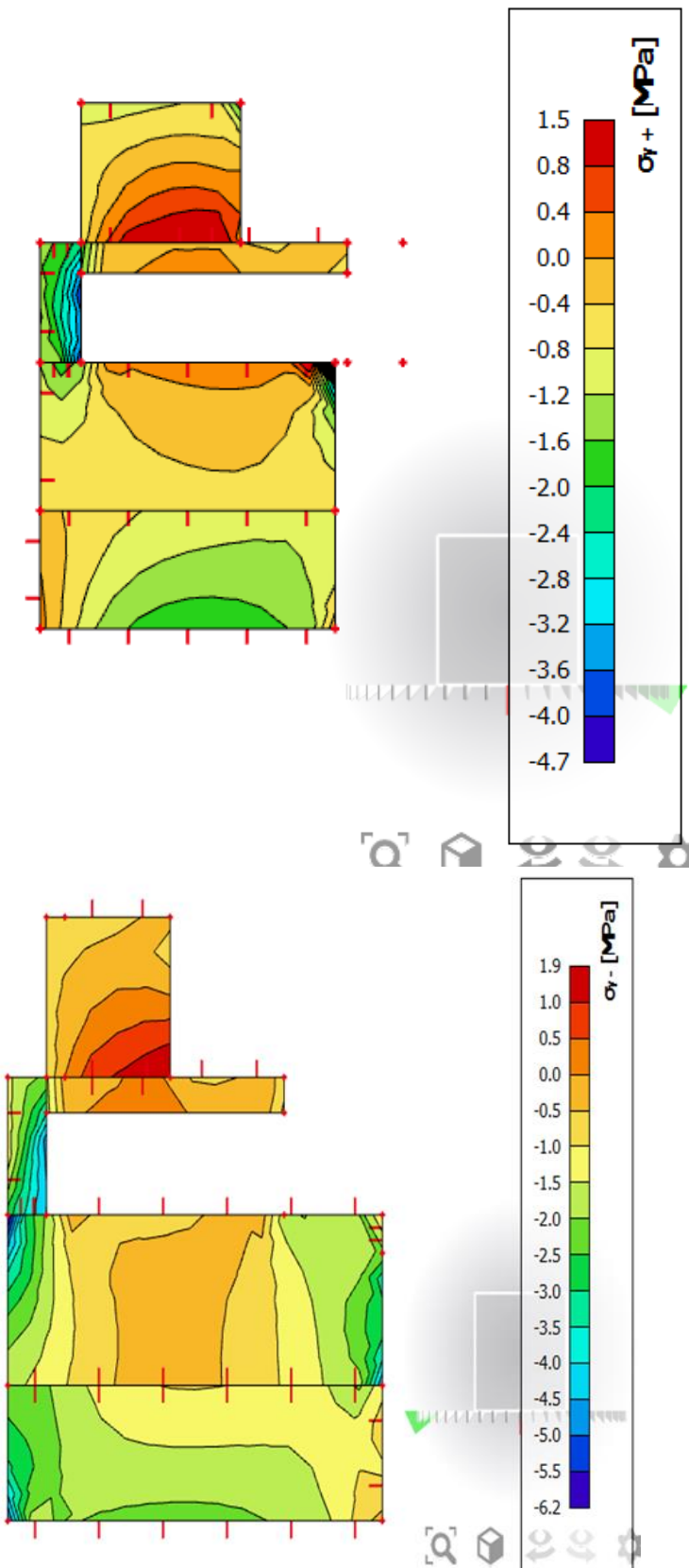
Slika 8.19. Naprezanja u smjeru y
