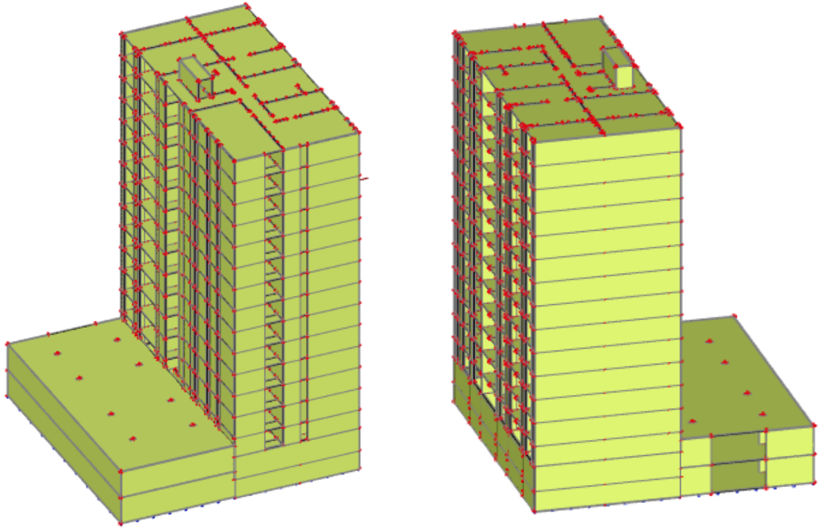
Slika 5.1. Numerički model
