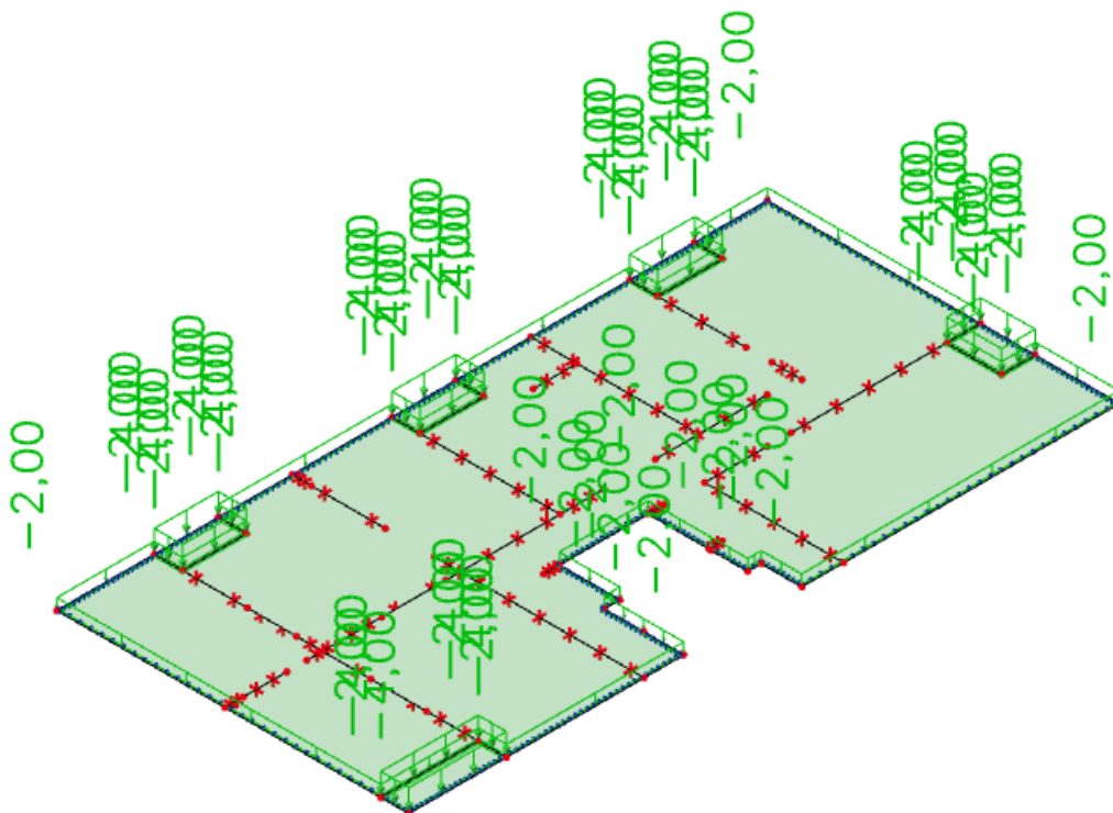
Slika 6.29. Korisno opterećenje (kN/m 2 )
