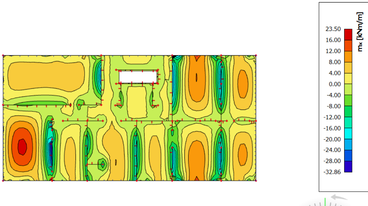
Slika 6.36. Maksimalni momenti savijanja M_x , za kombinaciju GSU
