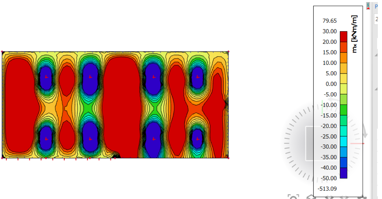
Slika 6.44. Prikaz momenata savijanja na ležajevima M_x – GSN1
