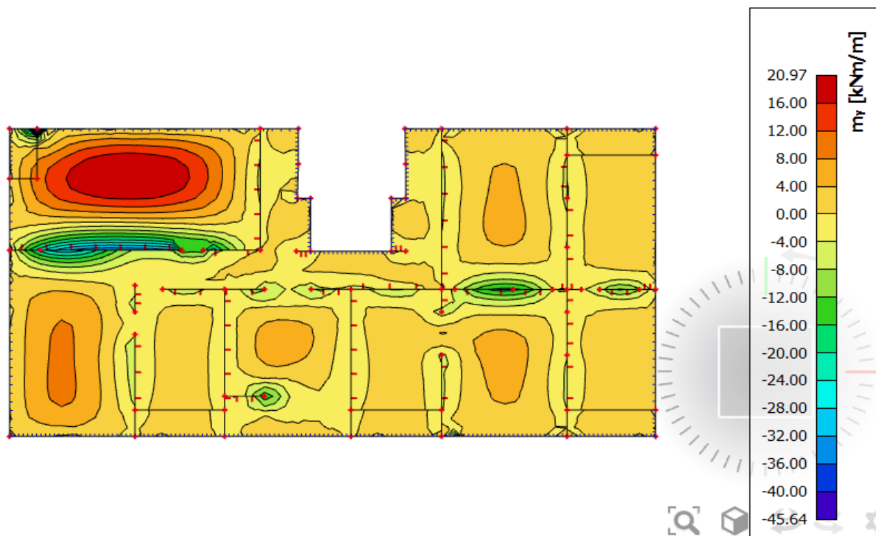
Slika 6.35. Maksimalni momenti savijanja M_y , za kombinaciju GSU
