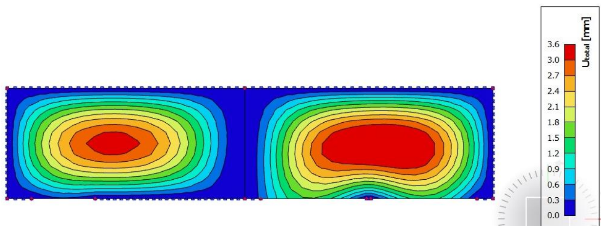
Slika 4.38. Prikaz progiba za ploču za kombinaciju GSU
