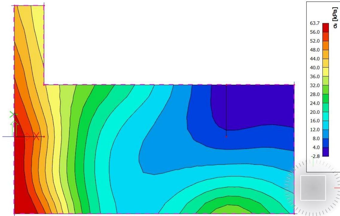
Slika 9.1. Kontaktna napreznja temeljne ploče 1
