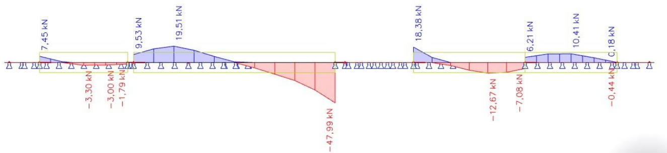
Slika 5.8. V_z (kN)
