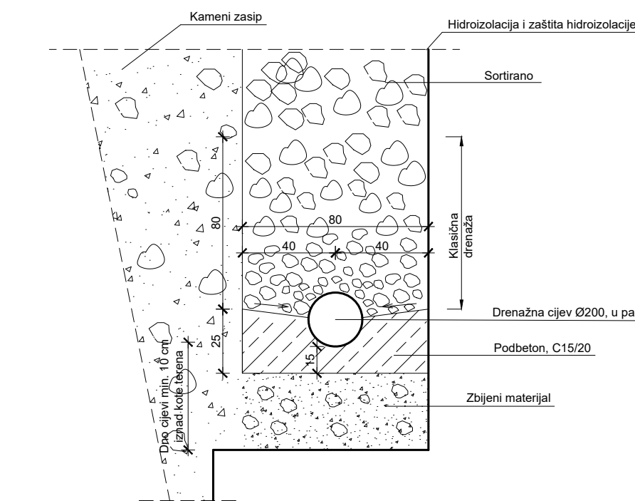
Detalj kanelura
