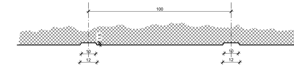
Detalj kanelura
