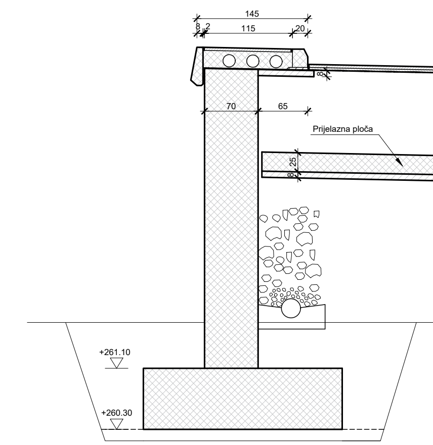
Presjek 7-7
