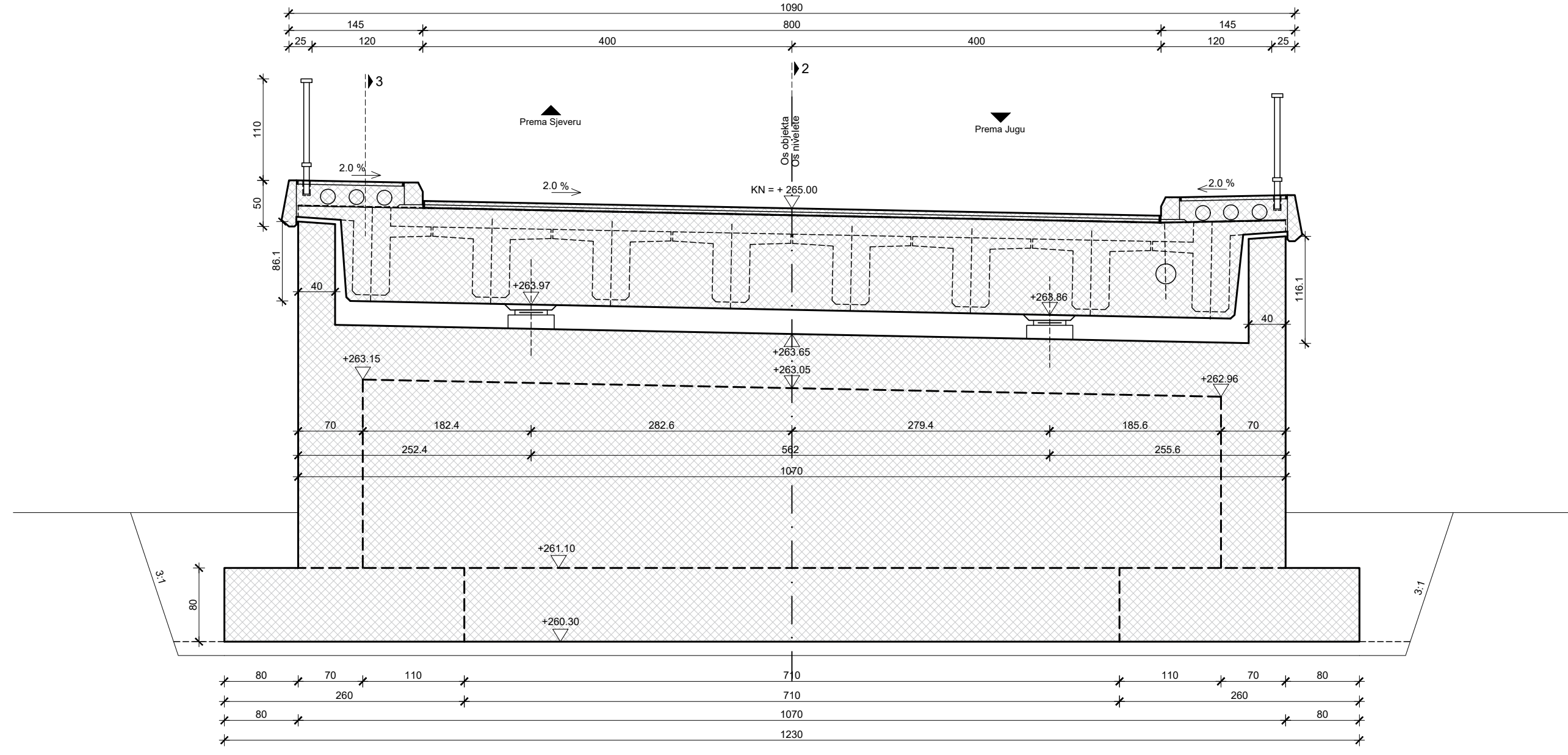
Presjek 1-1
