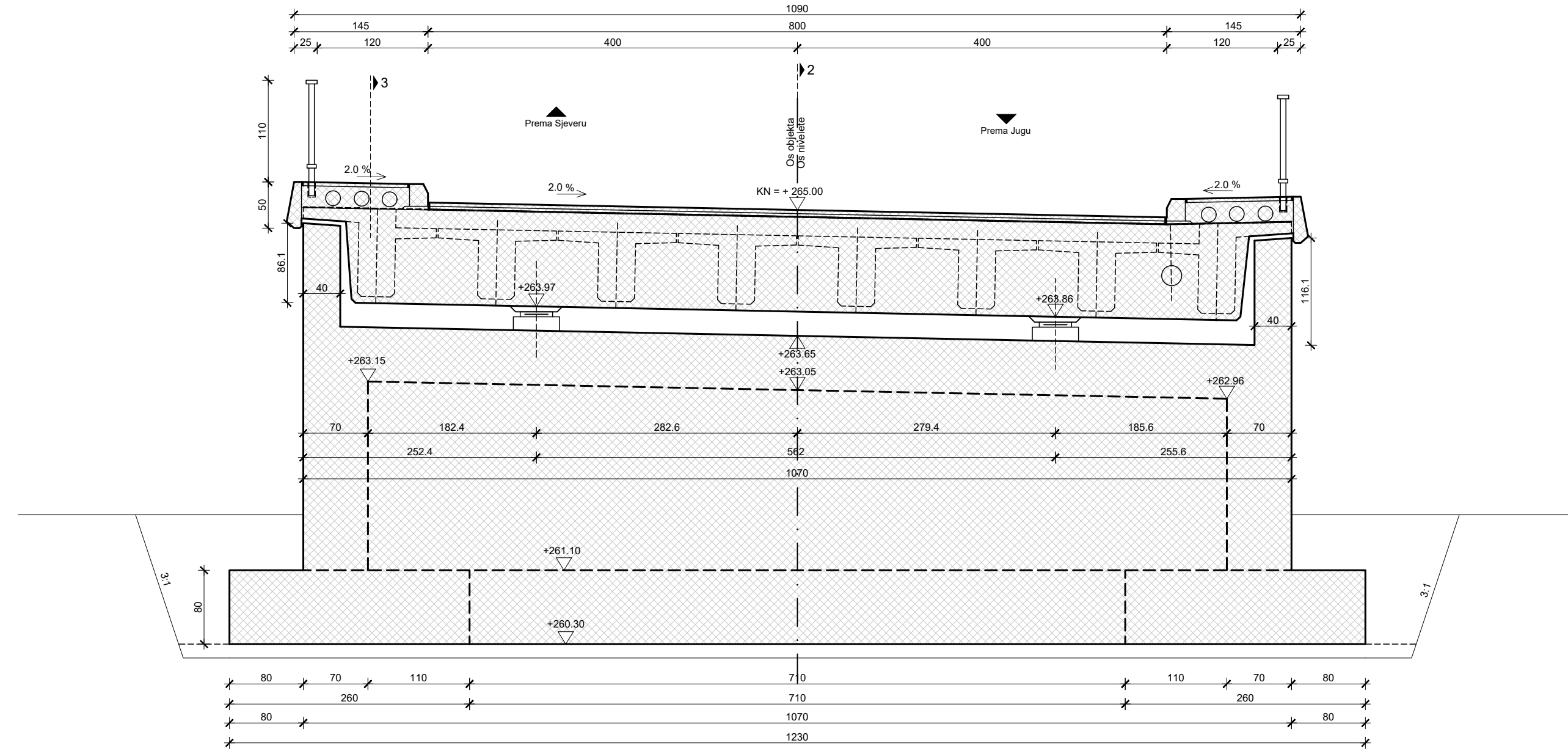
Presjek 1-1
