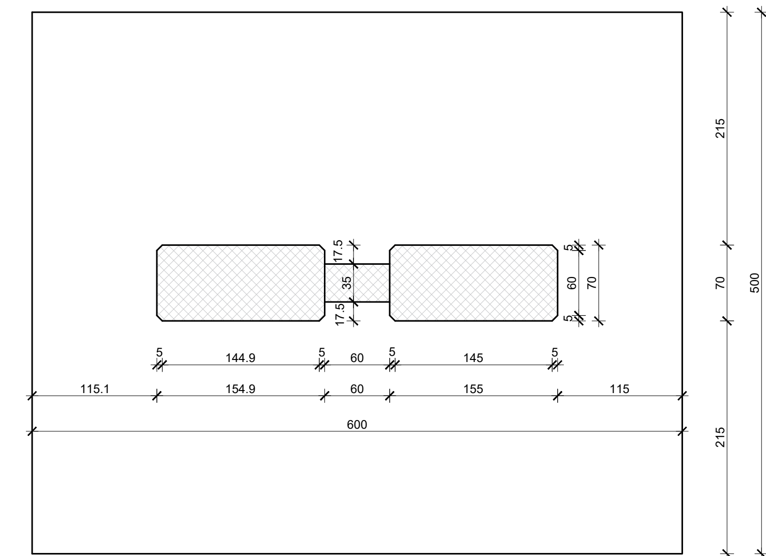
Presjek 4-4
