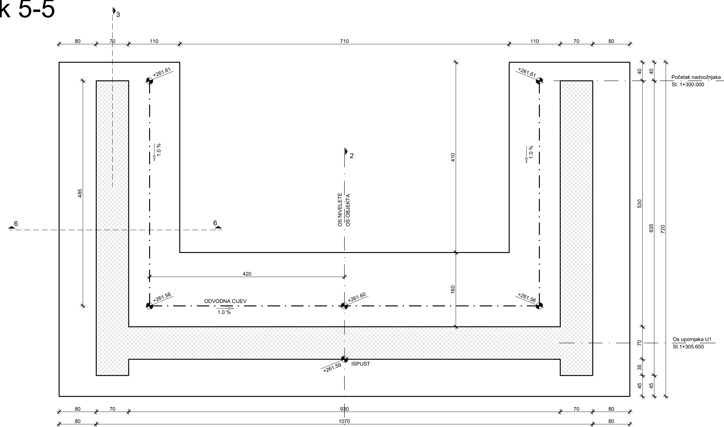
Presjek 6-6
