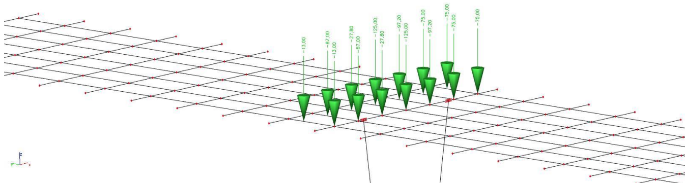
Slika 28: Prikaz tipskog vozila za maksimalnu poprečnu silu pri stupu
