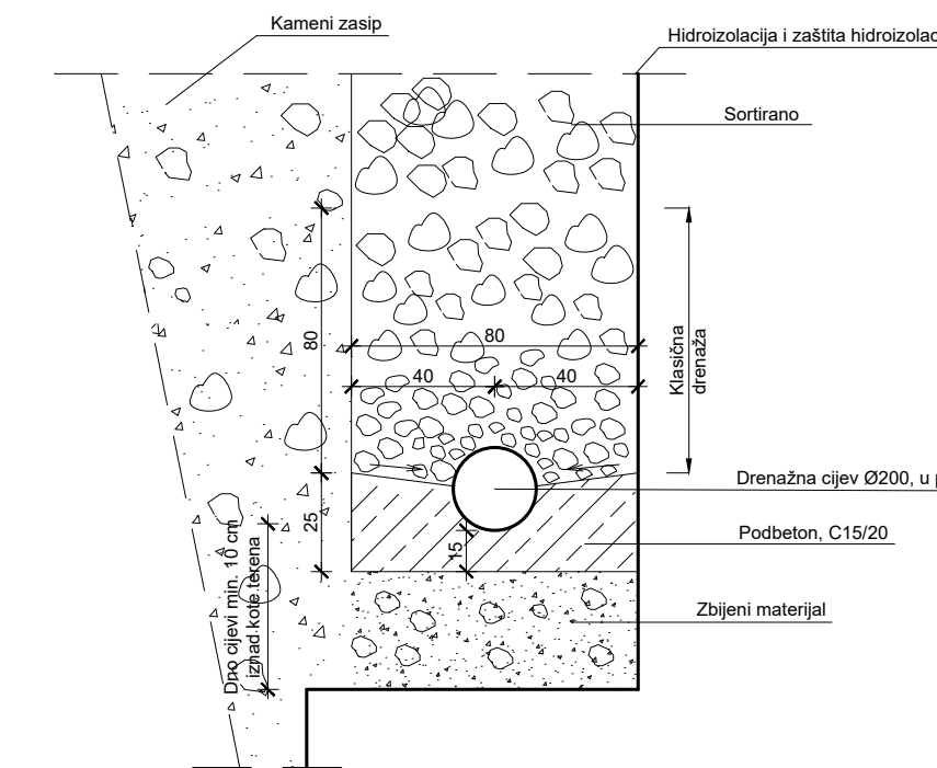
Detalj drenaže
