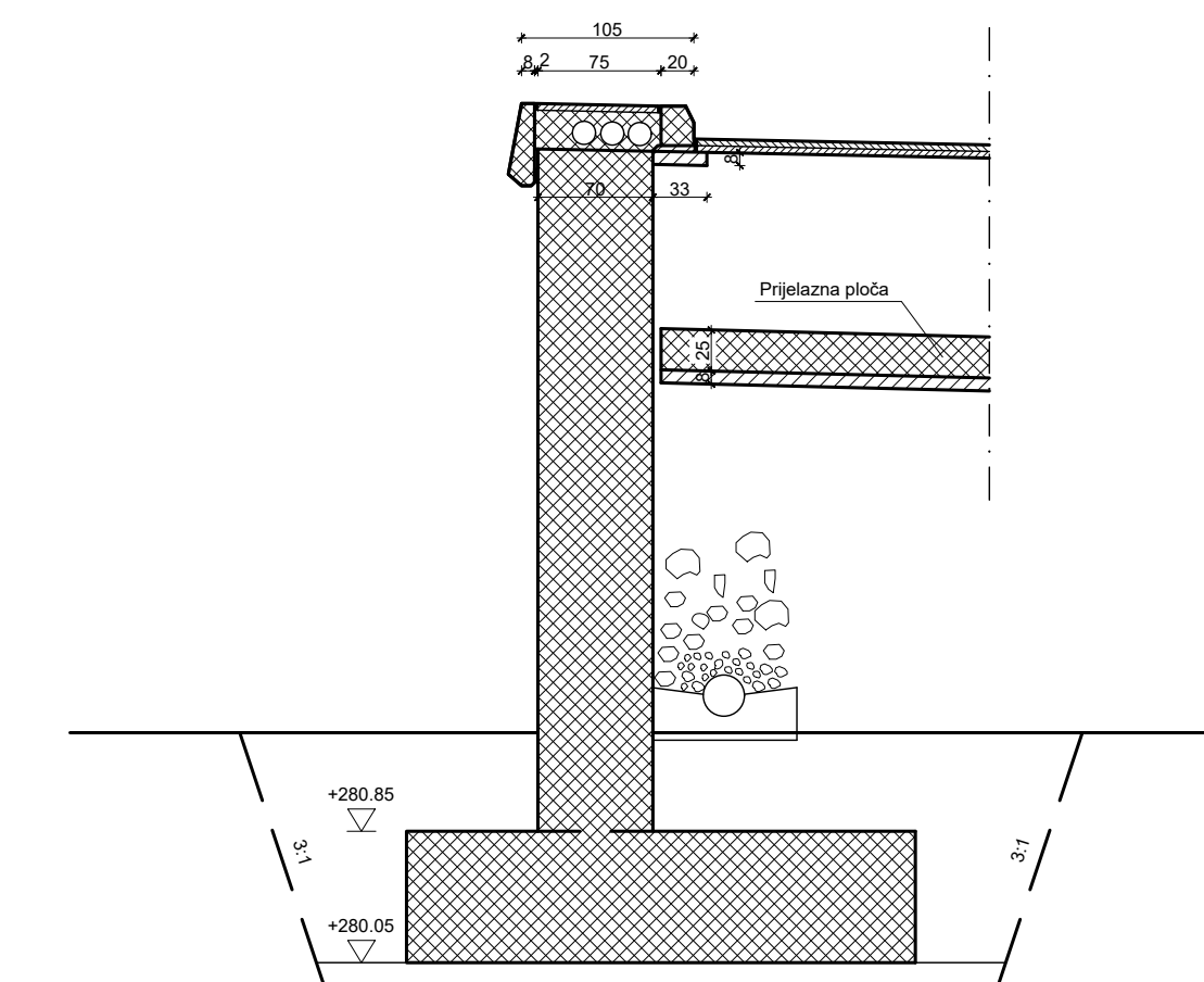
Presjek 7-7
