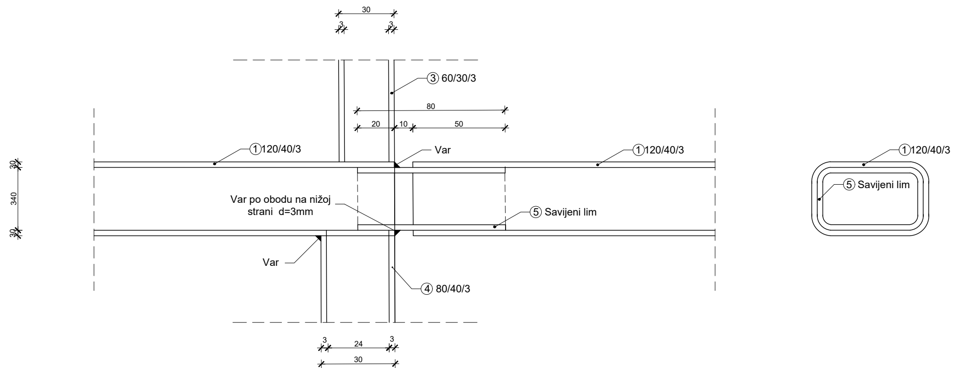
Detalj D 2 1:2
