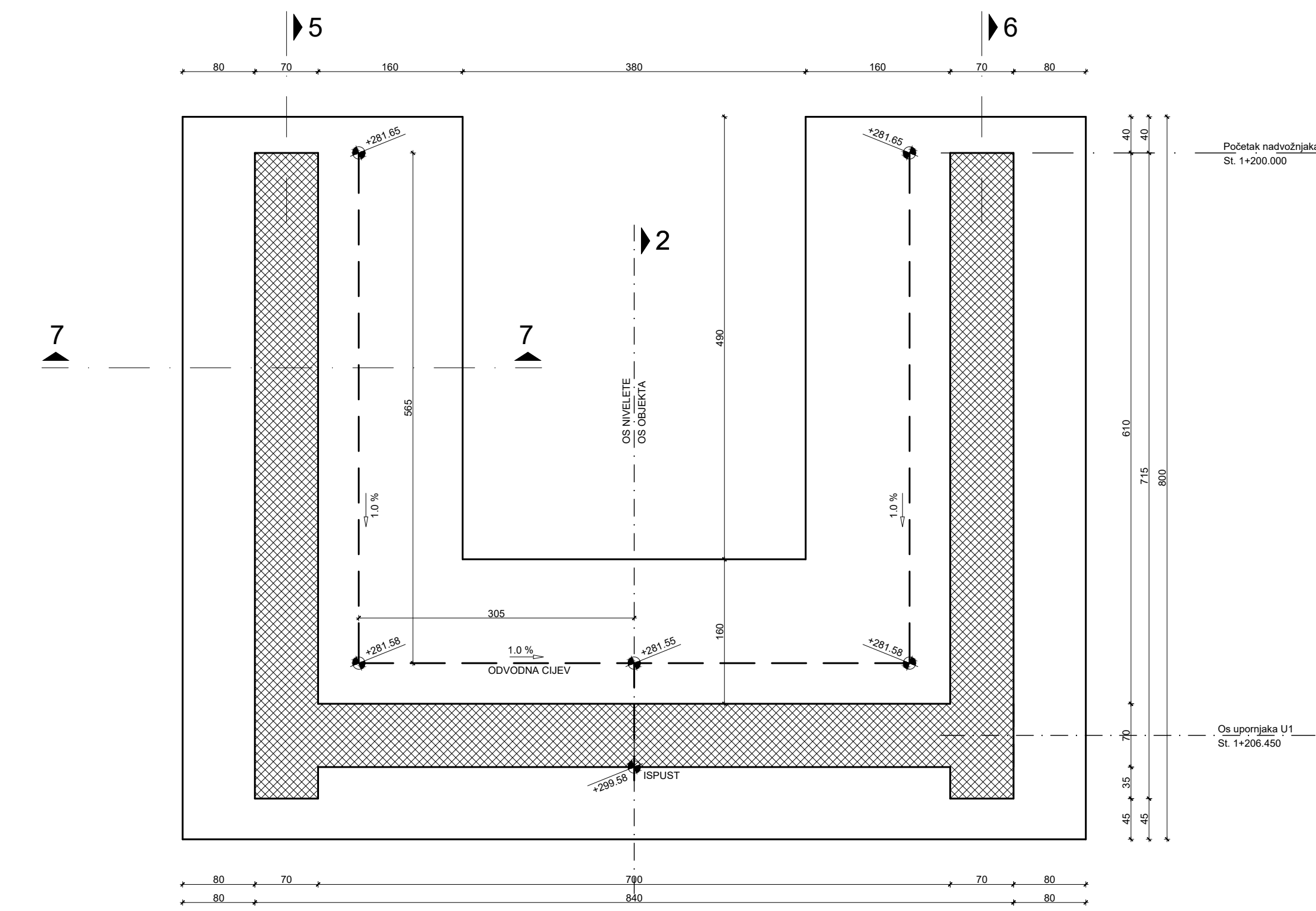
Presjek 3-3
