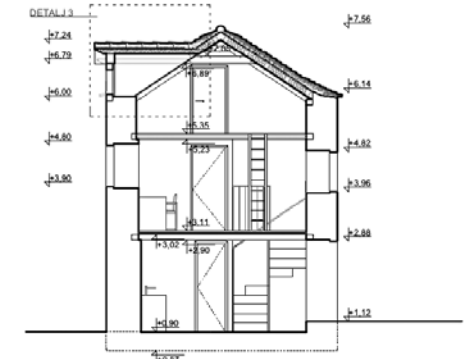
PRESJEK 2 - 2
