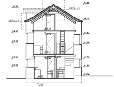
PRESJEK 1 - 1
