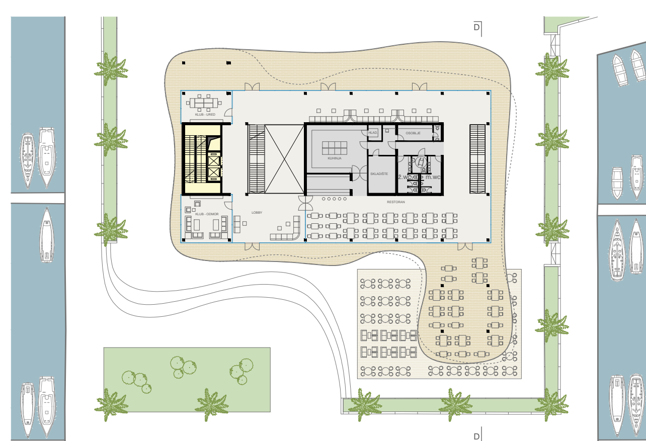
TLOCRT 1 KATA
