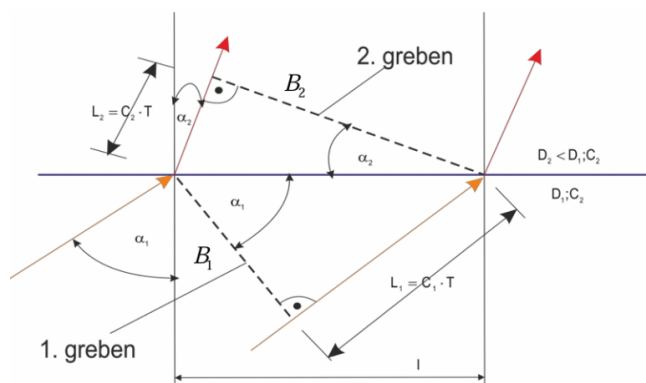
Slika 2.2 Snell-ov zakon
