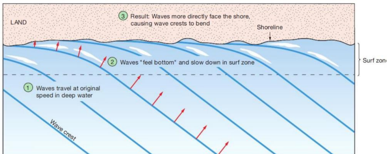
Slika 2. 4 Prikaz refrakcije.
