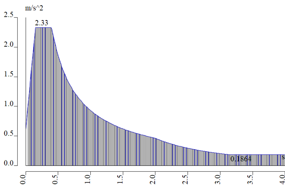
Slika 32. Proračunski spekter
